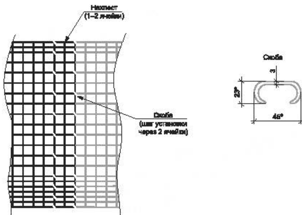
Рисунок В.1 — Устройство стыка смежных рулонов
