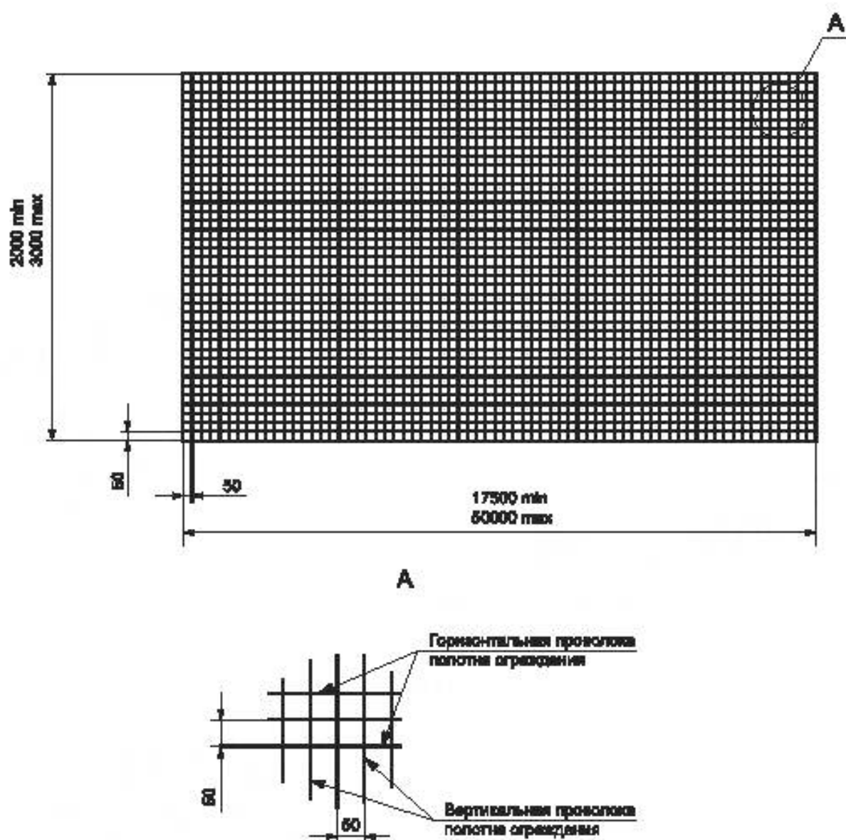
Рисунок Б.2 — Полотно ограждения с прямым профилем горизонтальной проволоки
