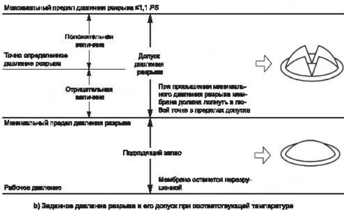
Рисунок 1 — Методы для определения разрывных мембран
