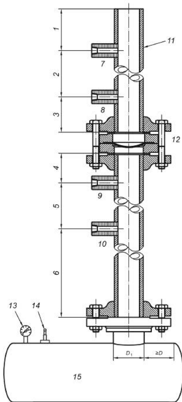
а) Принципиальная схема испытательного стенда
