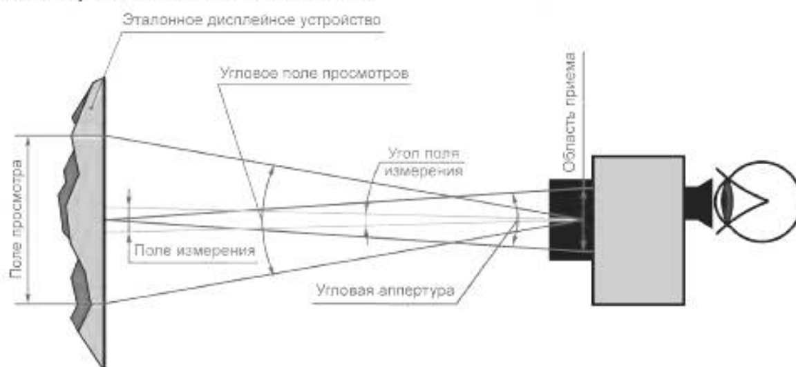
Рисунок 2 — Компонентная схема испытательной установки
