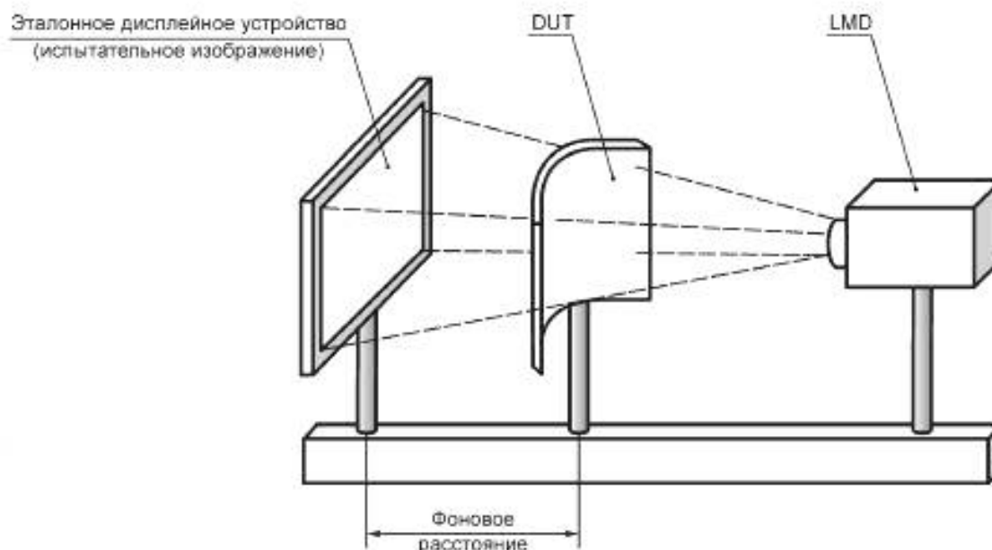
Рисунок 1 — Геометрическая конфигурация измерительной системы
