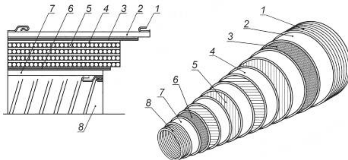
Рисунок 1 — Типовая конструкция гибкой трубы многослойной структуры со связующими слоями
