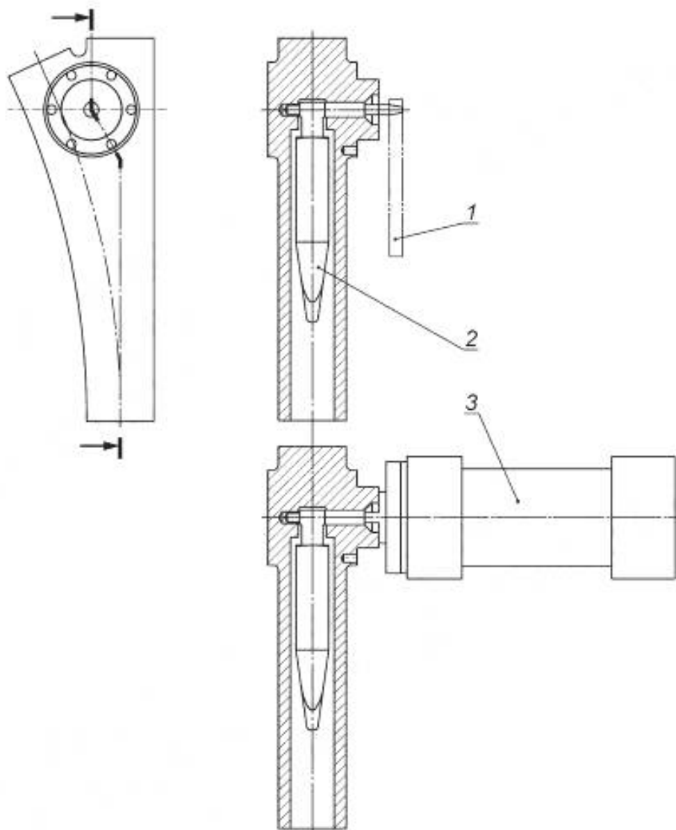
1 — внешняя рукоятка; 2 — лопасть дивертера; 3 — роторный привод
