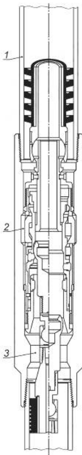
1 — колонка-носитель; 2 — захват паркинга; 3 — сервисная инструментальная колонна
