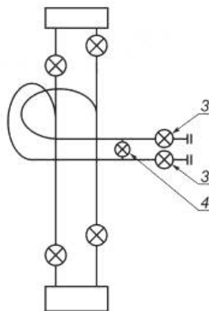
б) Схема альтернативной фонтанной арматуры системы TFL с перепускным клапаном до боковых задвижек (не распространена)
