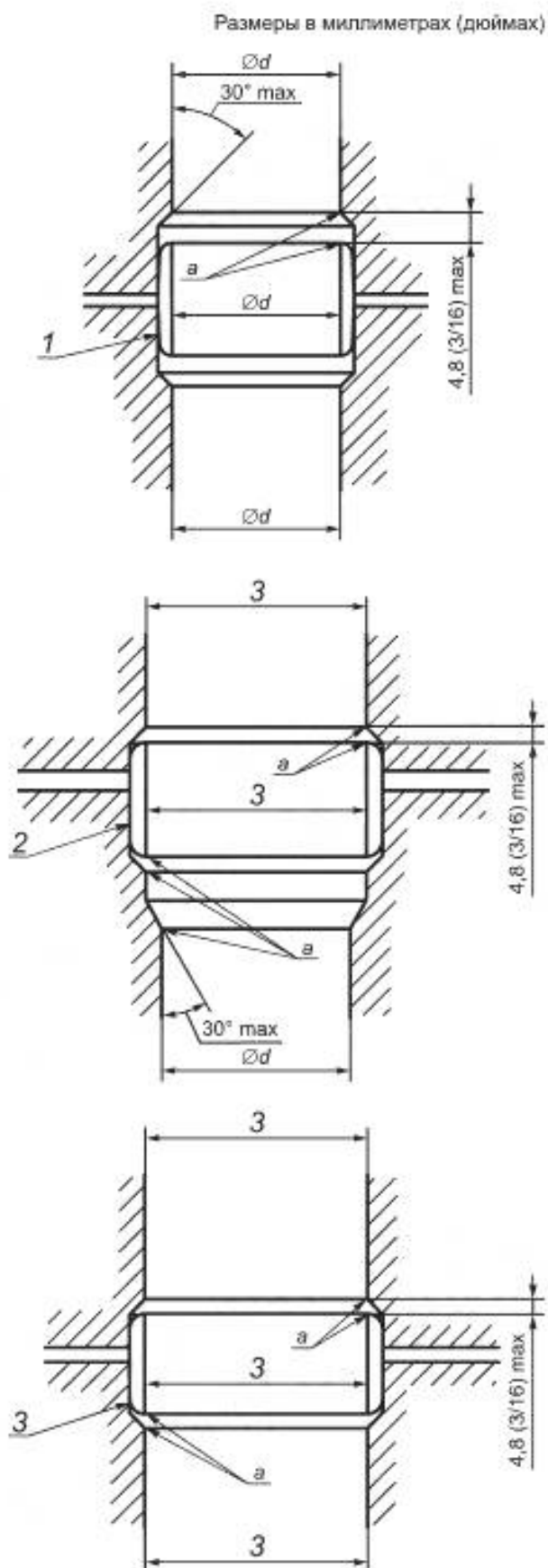
Рисунок 20 — Профили проходных отверстий с внутренними уплотнениями, лист 1
