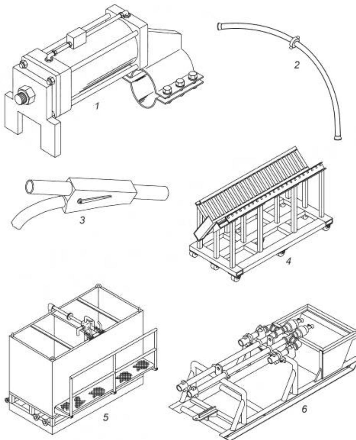
1 — гидравлическое устройство подачи инструмента; 2 — входные трубные летки; 3 — отводные устройства; 4 — ролик; 5 — рабочий резервуар; 6 — горизонтальный шлюз
