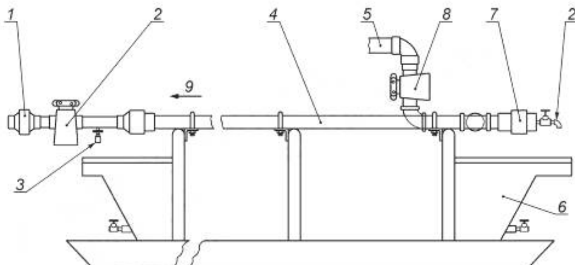
1 — быстросъемное соединение или фланец; 2 — отводящая арматура; 3 — полнопроходная трубопроводная арматура; 4 — труба увеличенного размера; 5 — трубопровод; 6 — сборники; 7 — глухая пробка с быстросъемным соединением; 8 — трубопроводная арматура; 9 — направление проводки инструмента
