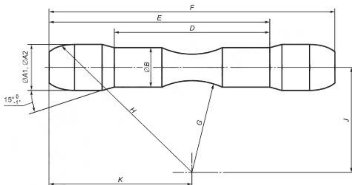
Рисунок 13 — Размеры контрольной оправки системы TFL
