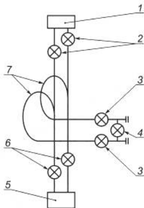
а) Схема типовой фонтанной арматуры системы TFL
