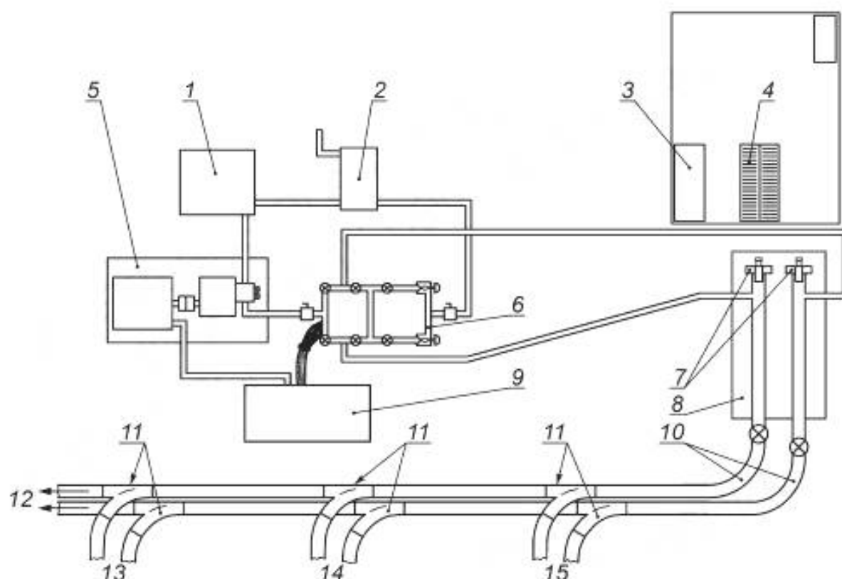
1 — смешительный резервуар для флюидов; 2 — резервуар для хранения; 3 — рабочий стол; 4 — ролпант; 5 — насосный блок; 6 — поверхностный управляющий manifold; 7 — устройства подачи инструмента; 8 — двойной горизонтальный шлюз; 9 — панель управления; 10 — входные трубные петли; 11 — отводные устройства; 12 — к другим скважинам в системе; 13 — скважина 3; 14 — скважина 2; 15 — скважина 1
