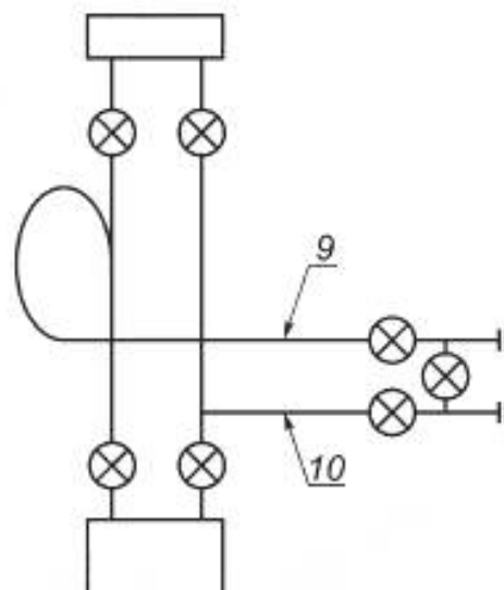
д) «Упрощенная» фонтанная арматура системы TFL
