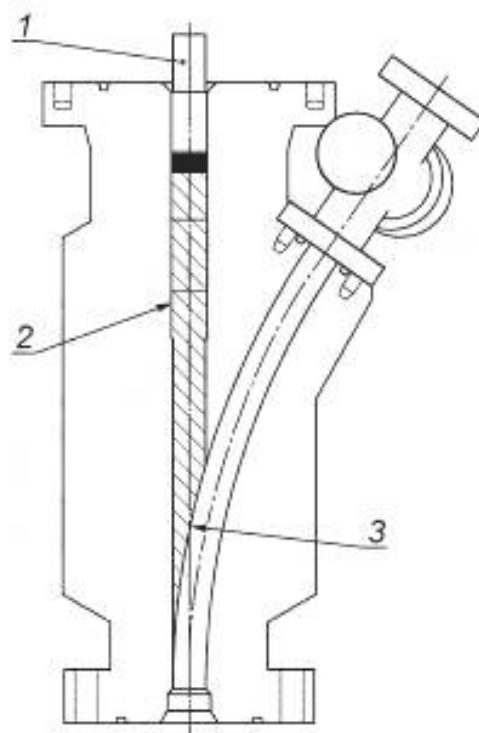
1 — профиль для извлечения с помощью каната; 2 — канатные внутренние профили и расточки для ориентации и блокирования клина в Y-образной катушке; 3 — клиновой контурный профиль
