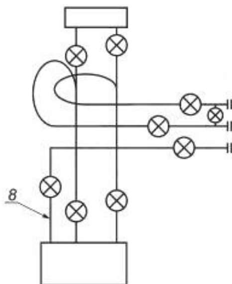
с) Фонтанная арматура TFL с отдельным доступом в затрубное пространство
