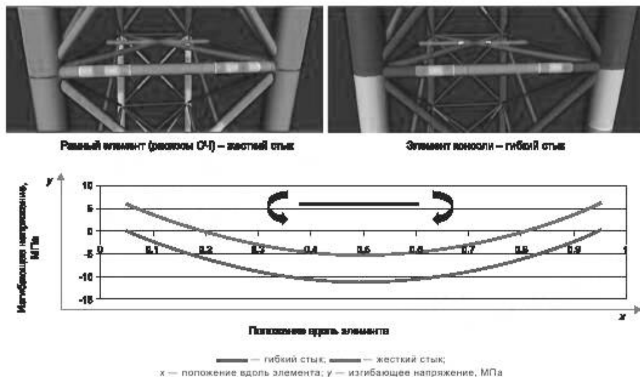
Рисунок А.3 — Изгибающее напряжение
