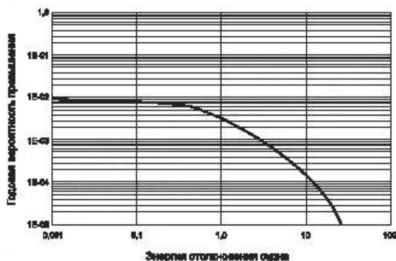
Рисунок А.11 — Пример кривой опасности столкновения судов
