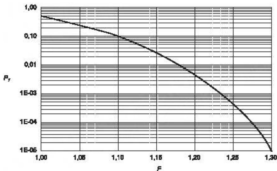
Рисунок А.8 — Пример кривой гравитационной опасности
