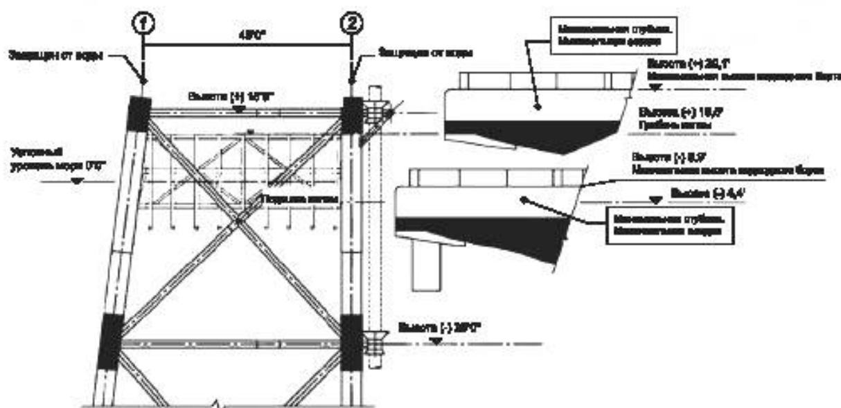
1, 2 — координатные оси основных стоек ОЧ
