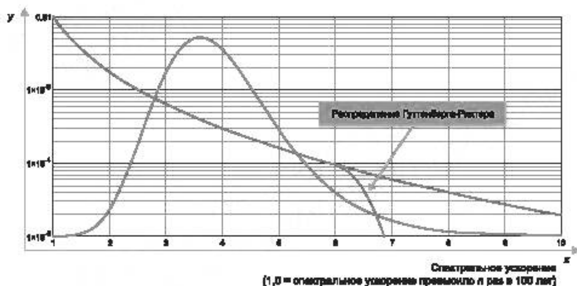
Рисунок А.10 — Пример кривой сейсмической опасности
