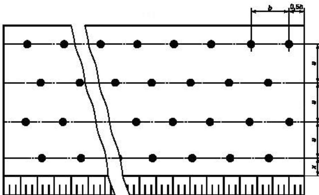
Рисунок 4 — Шестирядное расположение скважин
