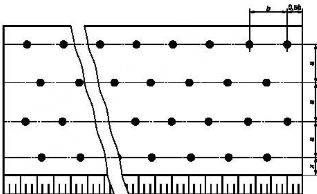
Рисунок 3 — Четырехрядное расположение скважин
