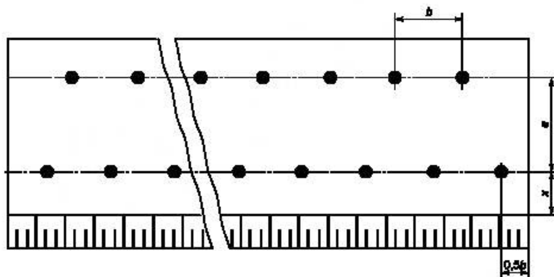
Рисунок 2 — Двухрядное расположение скважин
