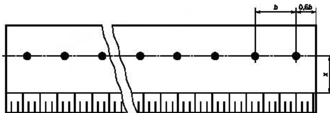
Рисунок 1 — Однорядное расположение скважин
