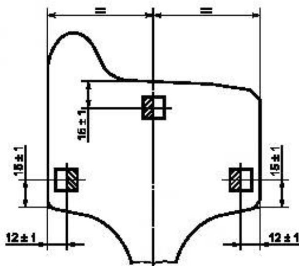
Рисунок 5 — Положение образцов для испытания на ударный изгиб в ободу колеса
