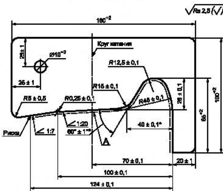
Рисунок А.1 — Профиль обода колеса
