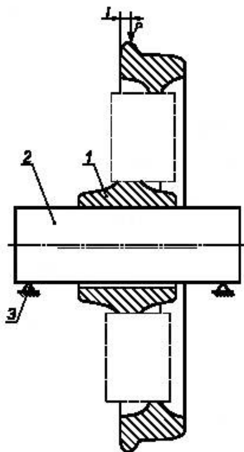
1 — колесо; 2 — ось; 3 — неподвижные опоры испытательной машины
