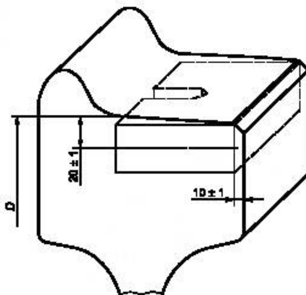
Рисунок 9 — Положение образца для определения трещиностойкости стали обода
