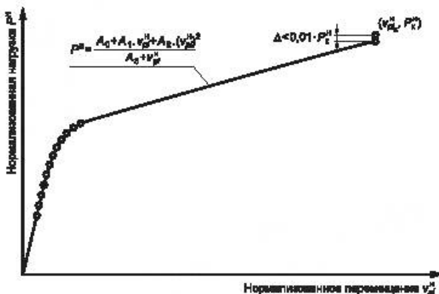
Рисунок K.4 — Аппроксимация нормализованной диаграммы уравнением (Л.7)
