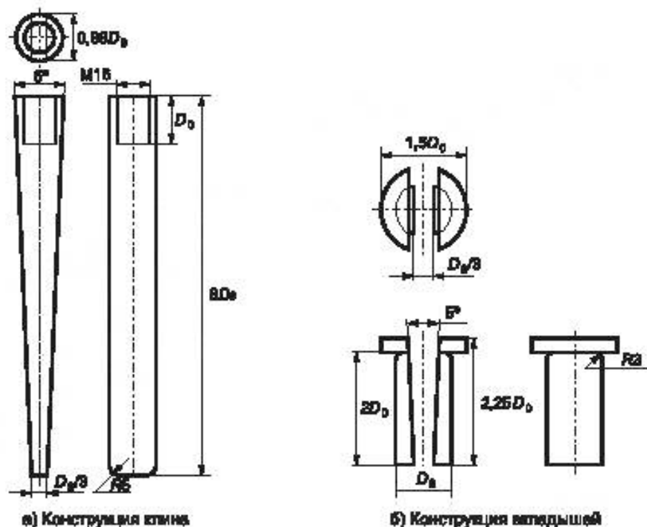
Рисунок 7.4 — Конструкция клина и вкладышей для испытаний образца типа ССА
