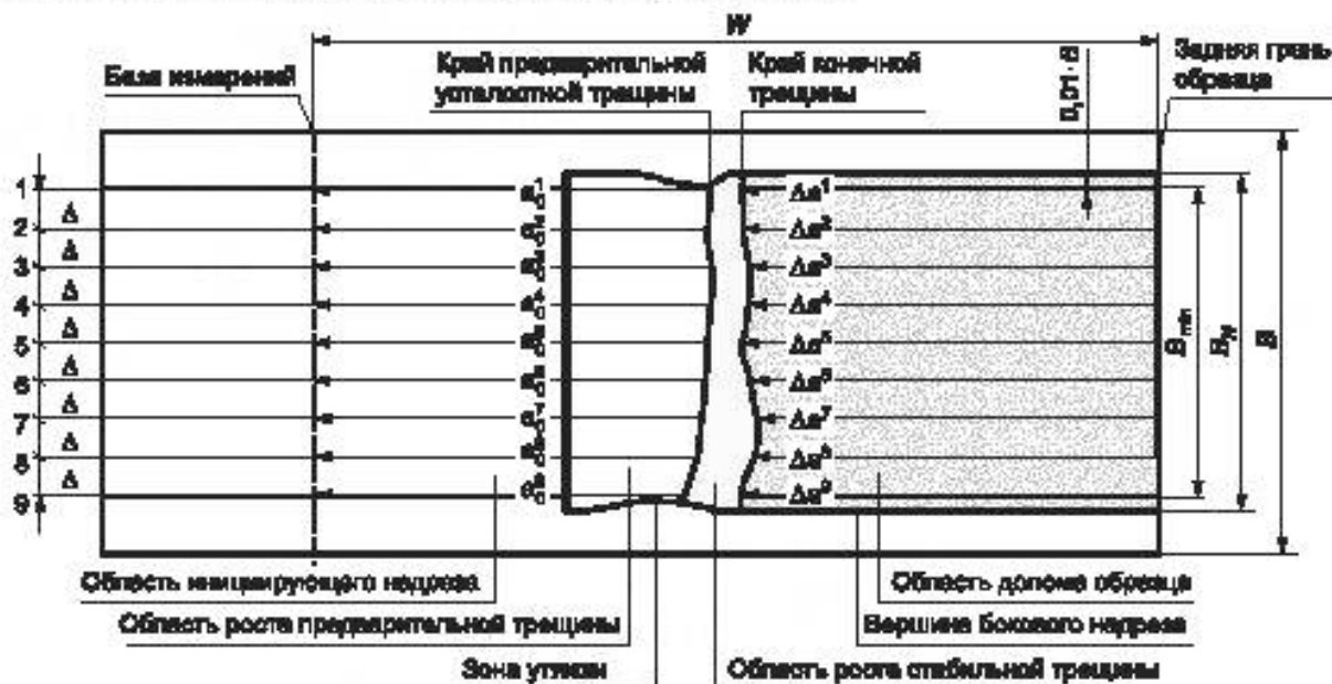
Рисунок Ж.1 — Схема определения длины предварительной усталостной трещины и величины стабильного подраста трещины для образцов типов CT, SE(B) и DT
