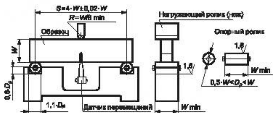
Рисунок 7.2 — Приспособление для установки образца типа SE(B)
