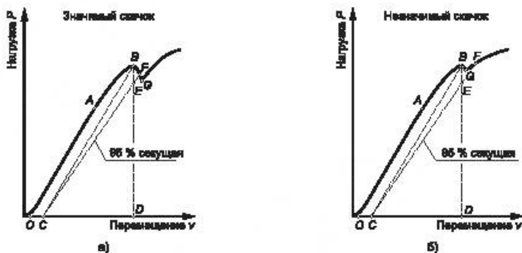
Рисунок И.1 — Оценка значимости скачка трещины
