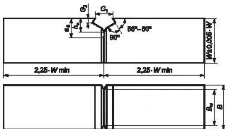
Рисунок Б.1 — Плоский прямоугольный образец типа SE(B)
