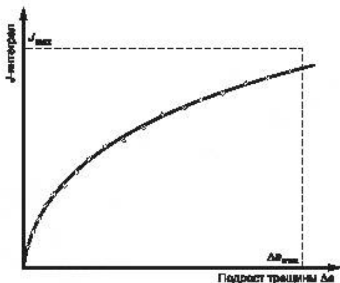
Рисунок 9.1 — Пример типичной J_R -кривой
