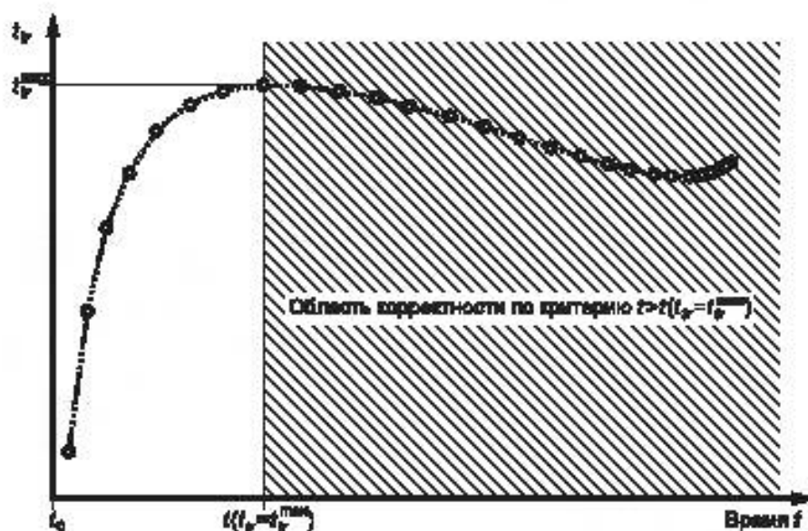
Рисунок 11.2 — Графическое представление критерия корректности по времени перехода к установившейся стадии ползучести
