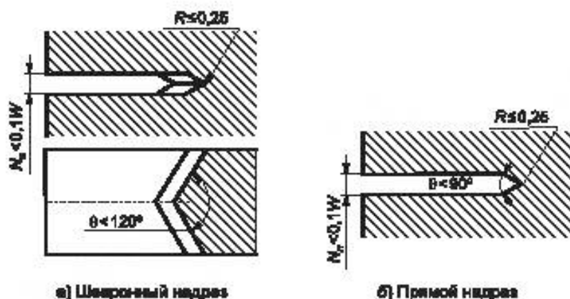
Рисунок 6.2 — Форма инициирующего надреза
