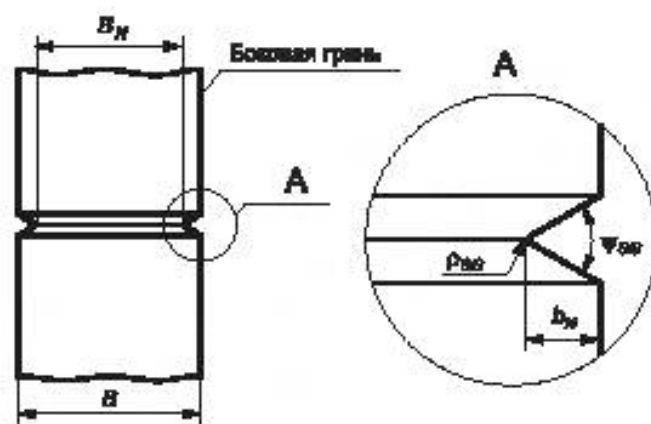
Рисунок 6.3 — Форма боковых канавок
