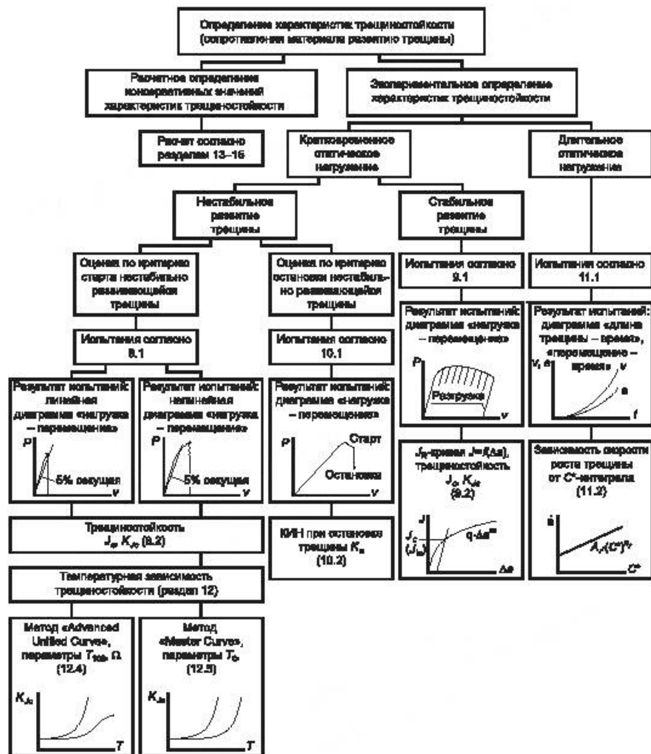
Рисунок 5.1 — Схема выбора методов и определения значений характеристик трещиностойкости материала
