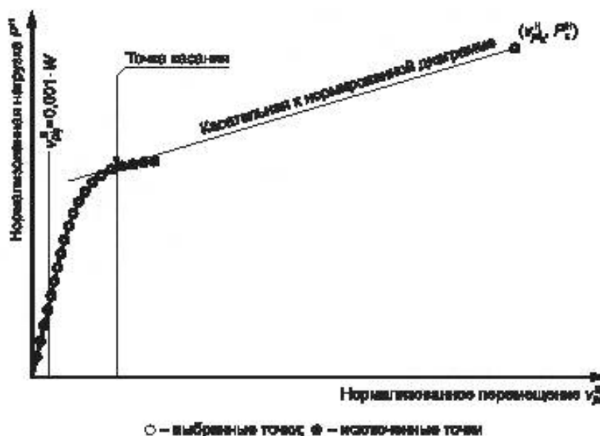
Рисунок К.3 — Выбор точек нормализованной диаграммы для дальнейшего анализа
