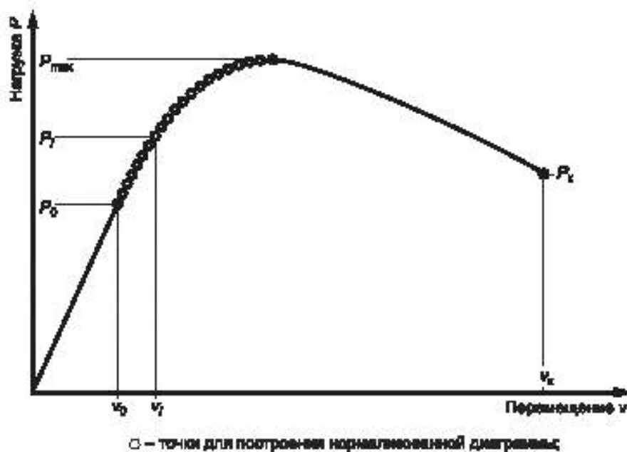
Рисунок К.1 — Диаграмма «нагрузка — перемещение по линии действия силы» и выбор точек на ней для построения нормализованной диаграммы
