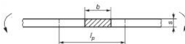
Рисунок 5.2 — Рабочая часть образца для испытаний при чистом изгибе
