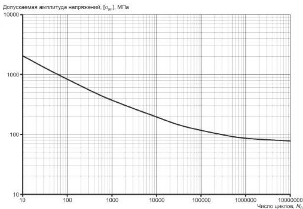
Рисунок А.1 — Расчетная кривая усталости материалов из углеродистых и легированных сталей ( R_{m0.2}^T/R_m^T \leq 0,7 , R_m^T \geq 460 МПа, Z^T \geq 32\% и E^T \geq 175 ГПа) в интервале температур от 20 °С до 350 °С
