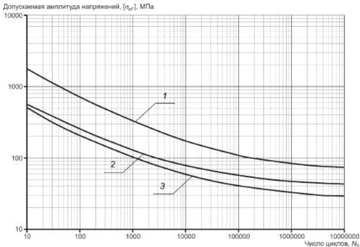
Рисунок А.8 — Расчетные кривые усталости материалов из сплава циркония с 2,5 % ниобия при длительности нагружения 2 \cdot 10^5 ч
