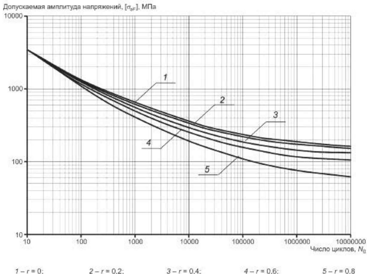
Рисунок А.4 — Расчетные кривые усталости для резьбовых участков шпилек и болтов из сталей перлитного класса с R_m^T \geq 760 МПа до температуры T = 350 °С при различных значениях коэффициента асимметрии r
