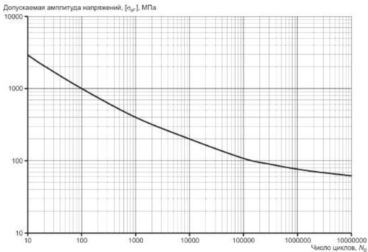
Рисунок А.2 — Расчетная кривая усталости материалов из сталей аустенитного класса ( R_{\text{ср}}^T/R_{\text{ср}}^T \leq 0,7 , R_{\text{ср}}^T \geq 360 МПа, Z^T \geq 45 % и E^T \geq 167 ГПа) в интервале температур от 20 °С до 450 °С
