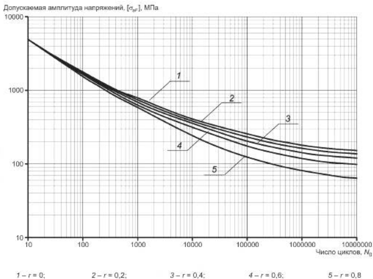
Рисунок А.3 — Расчетные кривые усталости для резьбовых участков шпилек и болтов из сталей перлитного класса с 660 \leq R_{\sigma T} < 760 МПа до температуры T = 350 °С при различных значениях коэффициента асимметрии r
