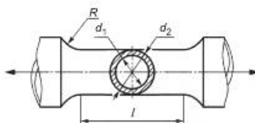
Рисунок 5.1 — Образец для испытаний при осевом растяжении-сжатии и кручении
