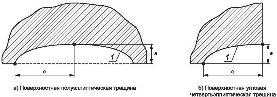
Рисунок 7.1 — Виды расчетного дефекта в компоненте
