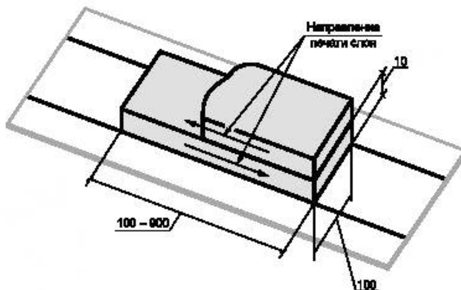
Рисунок 4 — Схема нанесения слоев при определении прокачиваемости
