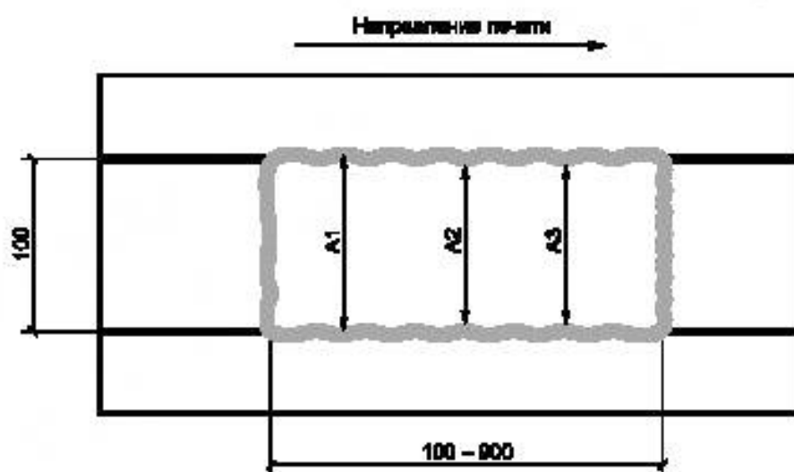
Рисунок 3 — Схема измерения оплыва нанесенного слоя
