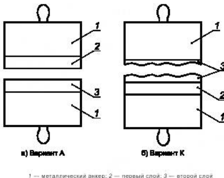
Рисунок 5 — Варианты разрушения образца при осевом растяжении
