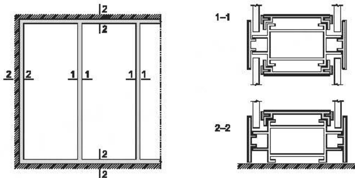
Рисунок А.4 — Двухслойная каркасная СвПП
