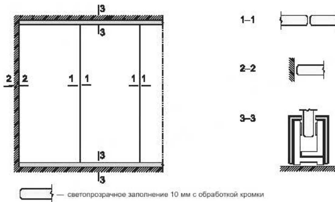
Рисунок А.5 — Однослойная цельностеклянная СвПП
