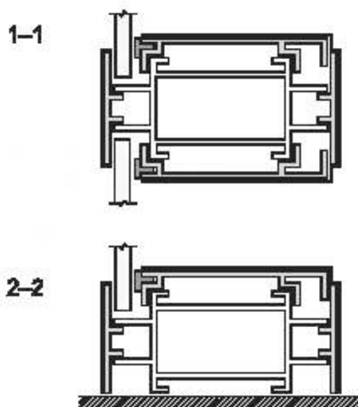
Рисунок А.3 — Однослойная каркасная СвПП с остеклением, расположенным по краю перегородки
