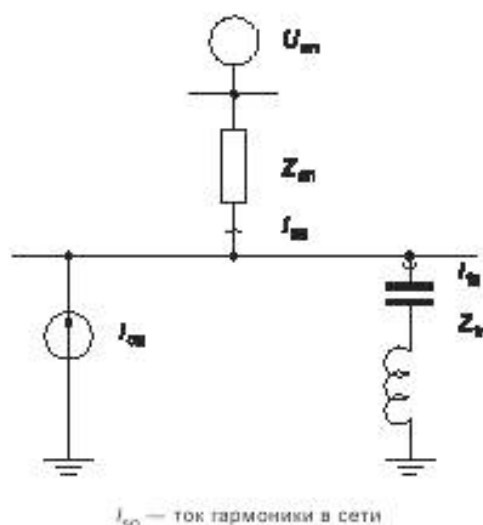
Рисунок 1 — Схема модели для оценки номинальных параметров элементов фильтра
