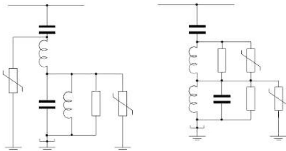
Рисунок 5 — Типовые варианты подключения ОПН
