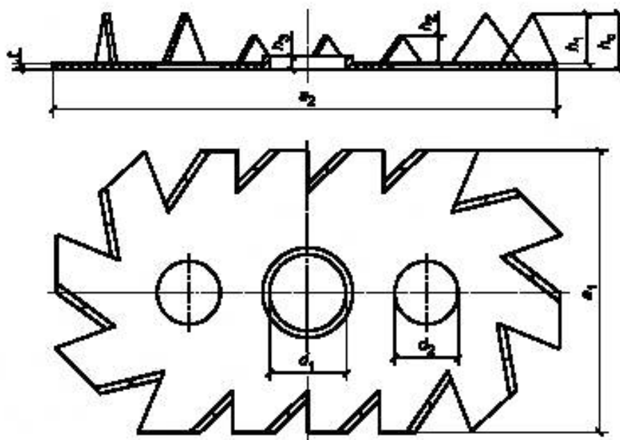
Рисунок А.4 — Зубчатая кольцевая шпонка типа С-4
