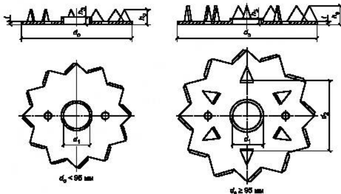
Рисунок А.2 — Зубчатая шпонка типа С-2
