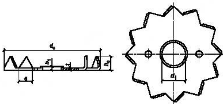
Рисунок А.7 — Зубчатая шпонка типа С-7
