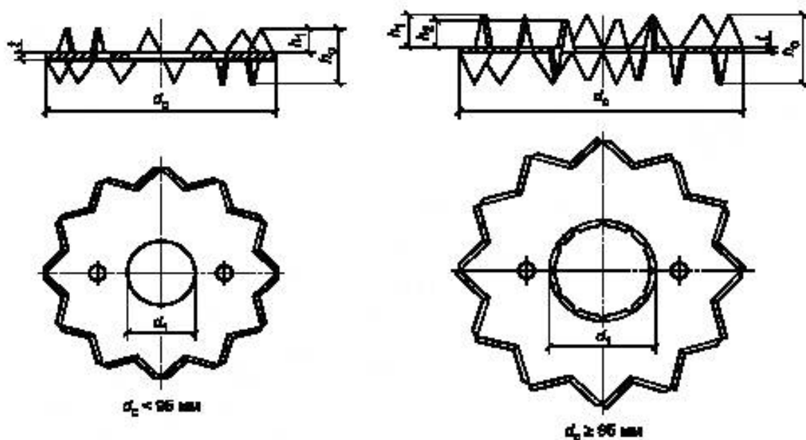
Рисунок А.1 — Зубчатая шпонка типа С-1
