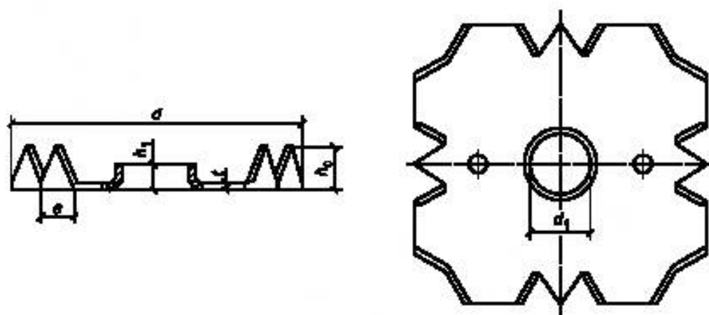
Рисунок А.9 — Зубчатая шпонка типа С-9
