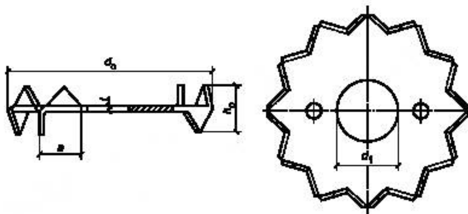
Рисунок А.6 — Зубчатая шпонка типа С-6
