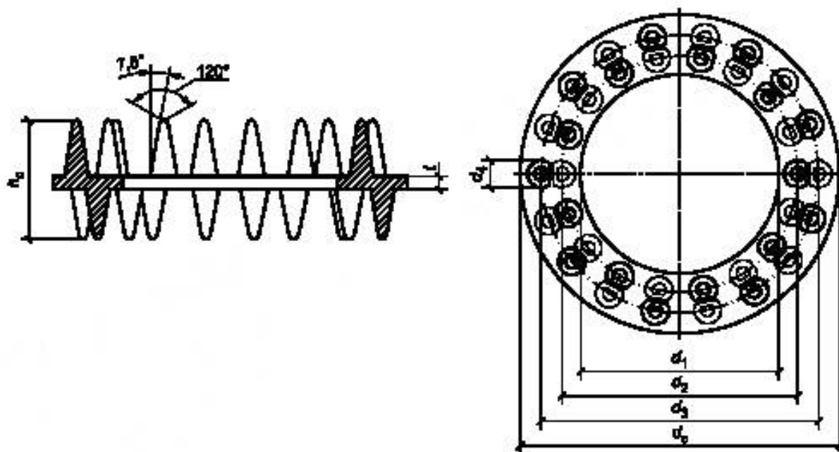
Рисунок А.10 — Зубчатая шпонка типа С-10
