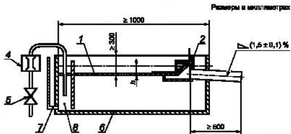
а) Паралетная воронка горизонтальная
