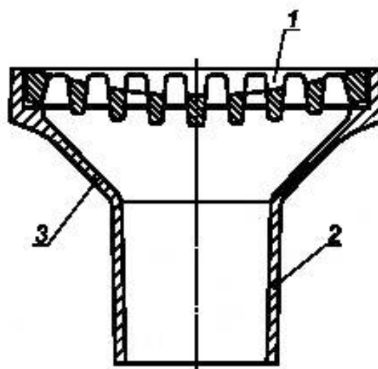
1 — решетка; 2 — выпускной патрубок; 3 — корпус трапа
