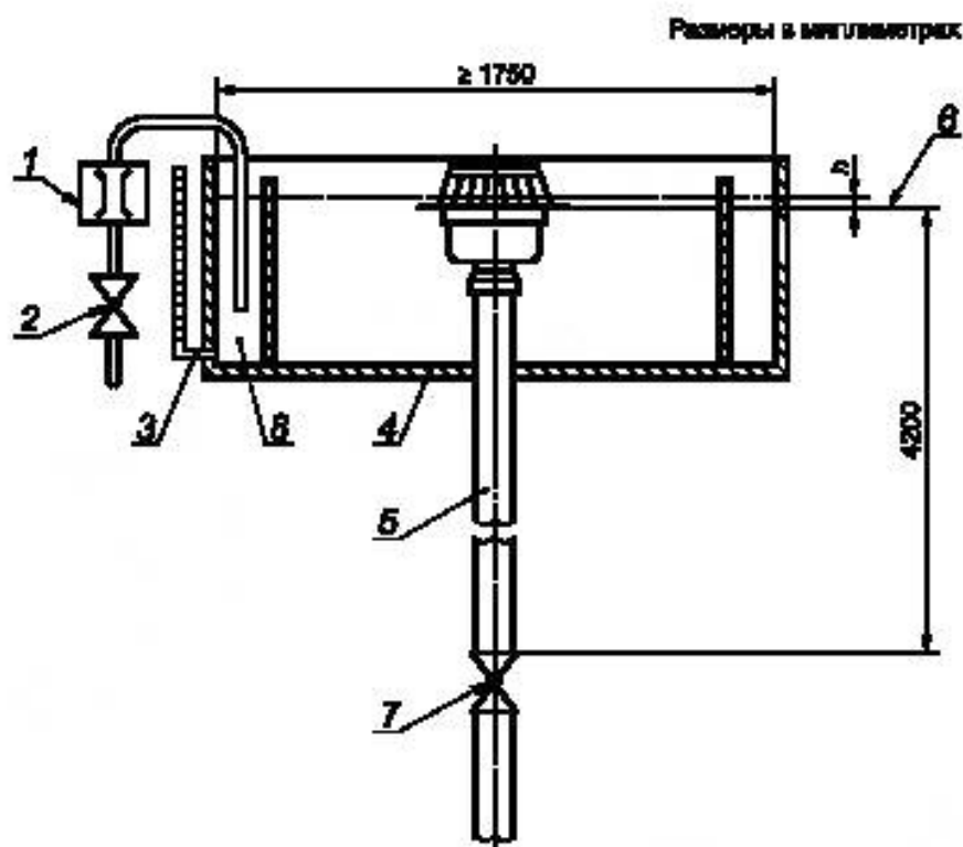
б) Кровельная воронка вертикальная
