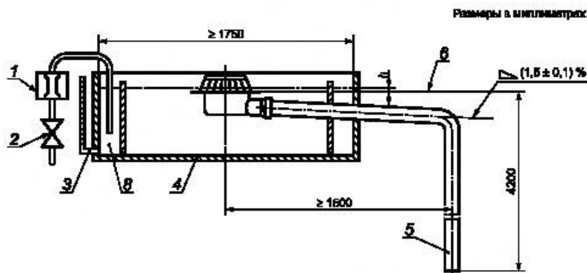
а) Кровельная воронка горизонтальная
