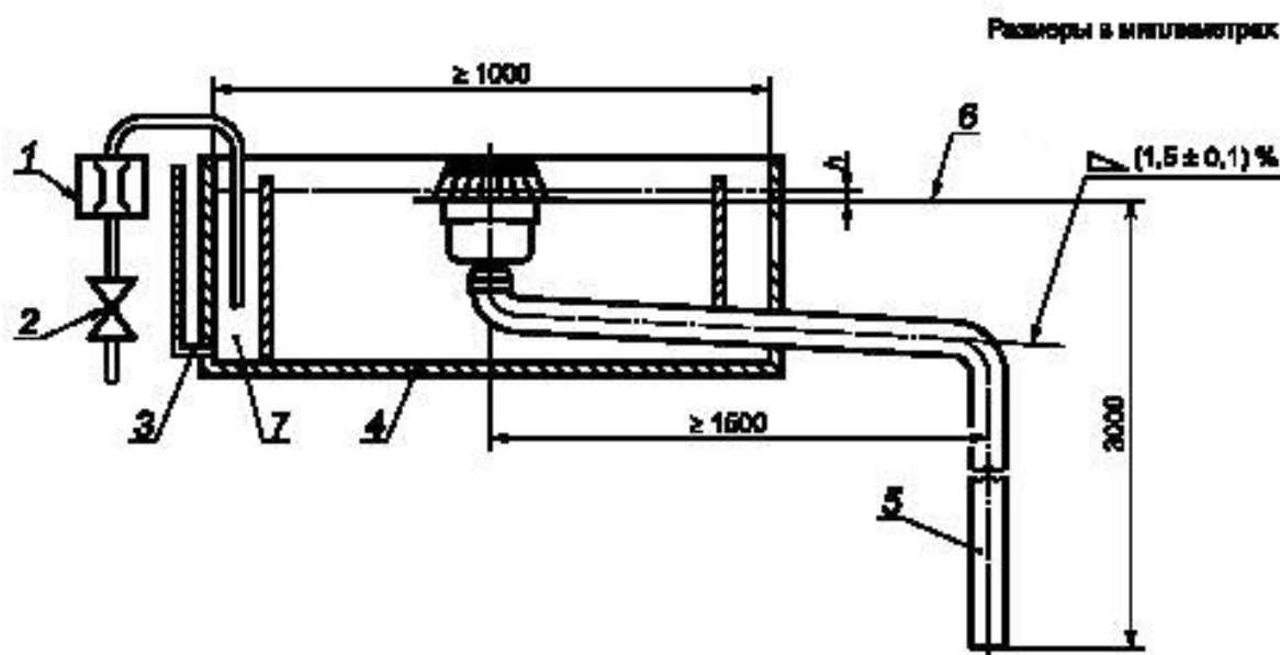
б) Кровельная воронка, вертикальная
