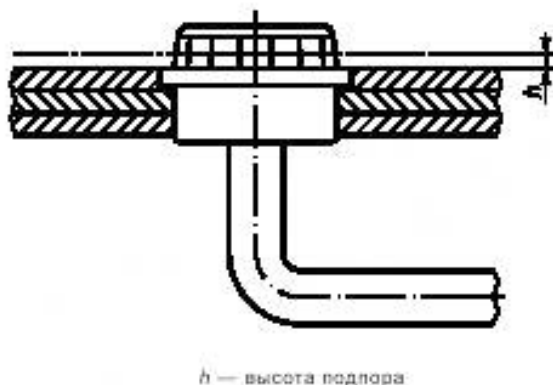
Рисунок 4 — Высота подпора
