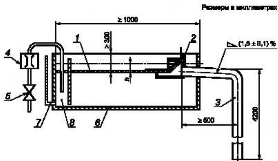
б) Паралетная воронка вертикальная
