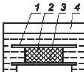
1 — сетчатый пригруз; 2 — образец; 3 — сетчатая подставка; 4 — ванна
