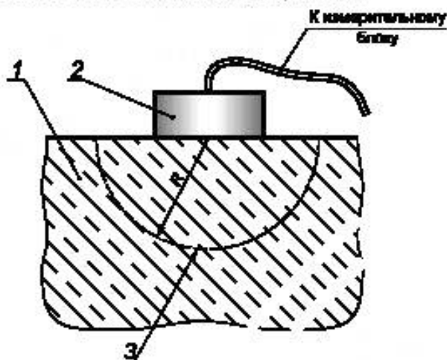
Рисунок 1 — Схема определения влажности поверхностным датчиком
