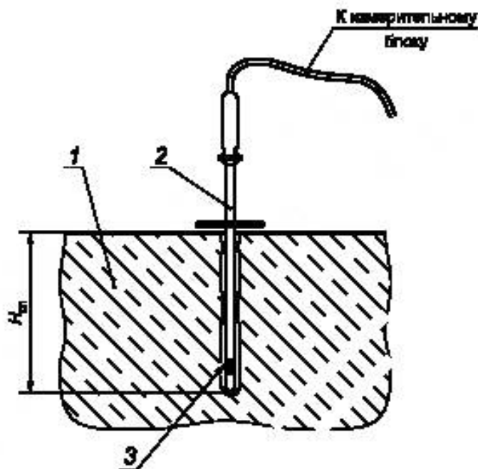
Рисунок 2 — Схема установки зондового датчика
