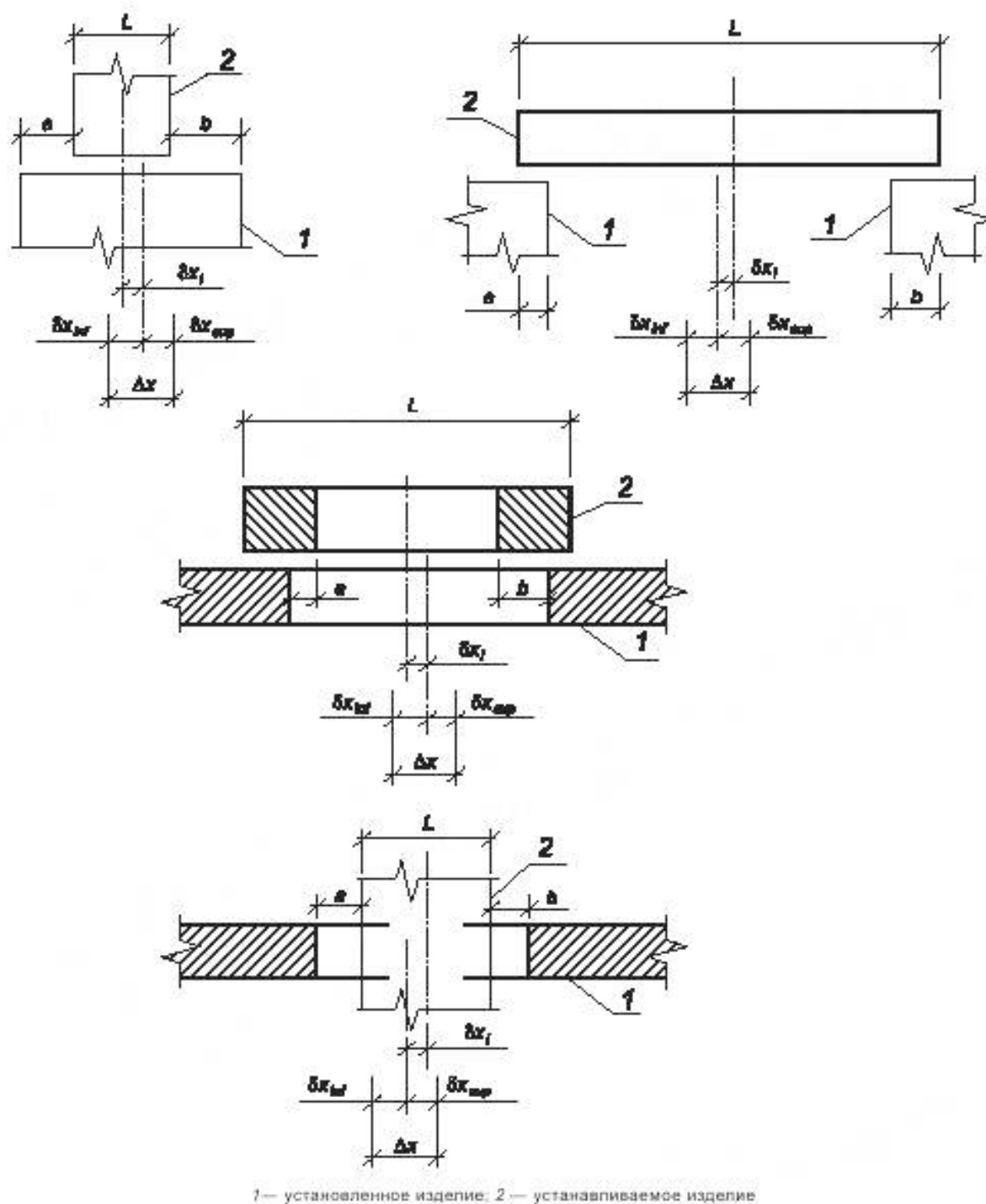
Рисунок 12 — Допуски симметричности и предельные отклонения точек поверхности от симметричности установки изделий
