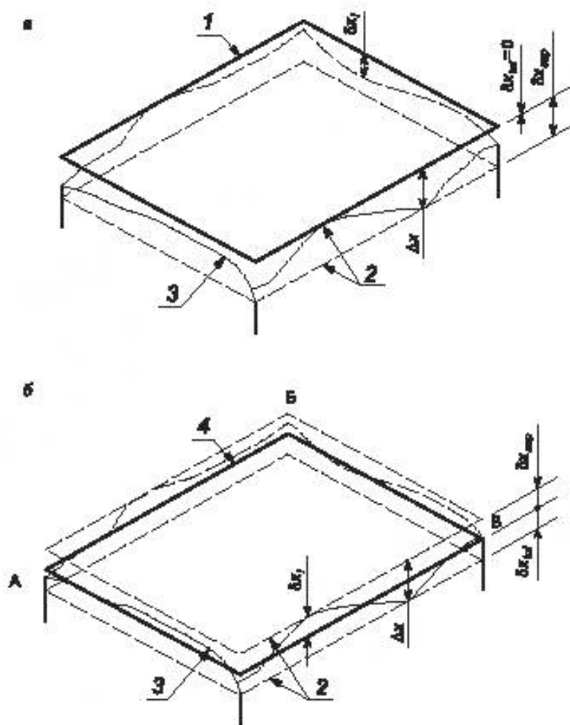
1 — условная (прилегающая) плоскость; 2 — плоскости, ограничивающие поле допуска; 3 — реальная поверхность; 4 — условная (проходящая через три крайние точки) плоскость; А — В — В — крайние точки реальной поверхности
