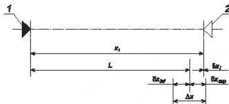
Рисунок 5 — Допуски и предельные отклонения разбивки точек и осей в плане
