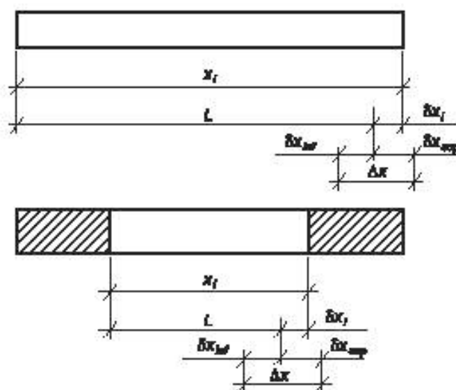
Рисунок 1 — Допуск и отклонение от линейных размеров изделий
