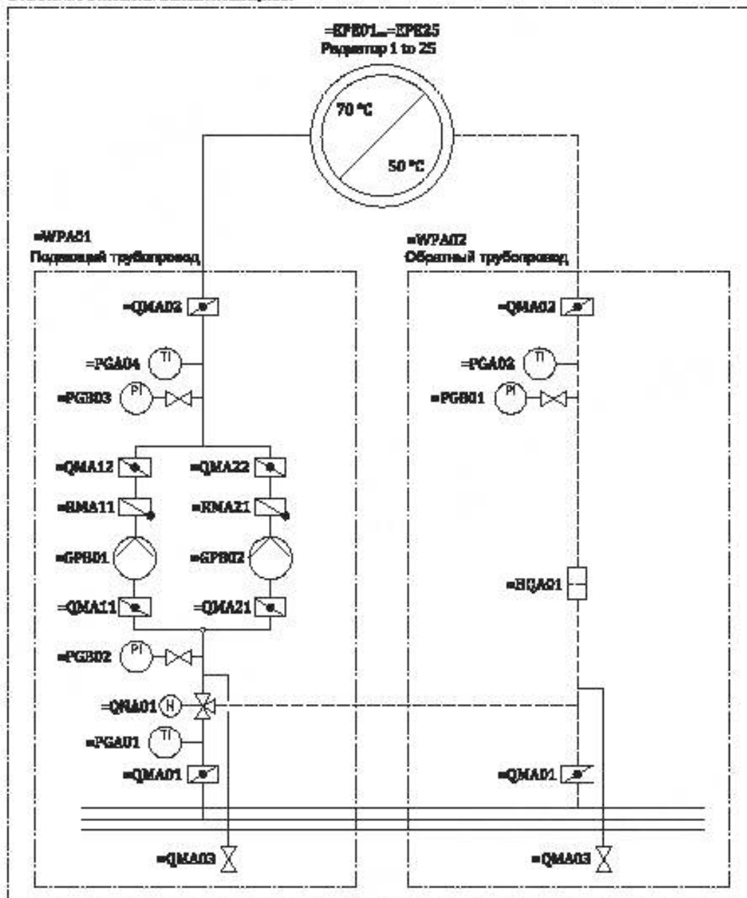
Рисунок В.17 — Принципиальная схема системы отопления
