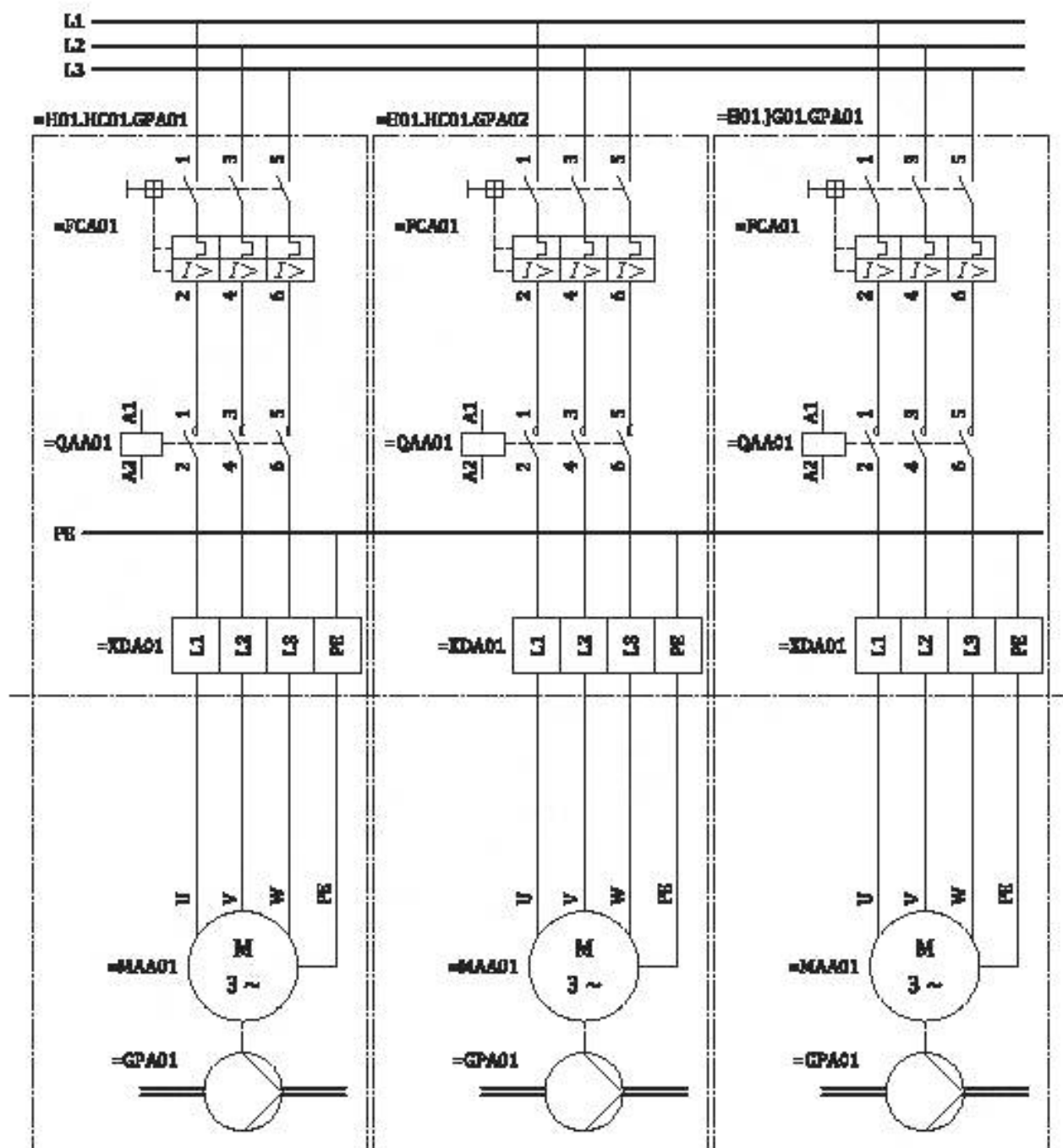
Рисунок В.23 — Схема электроснабжения трех насосных установок
