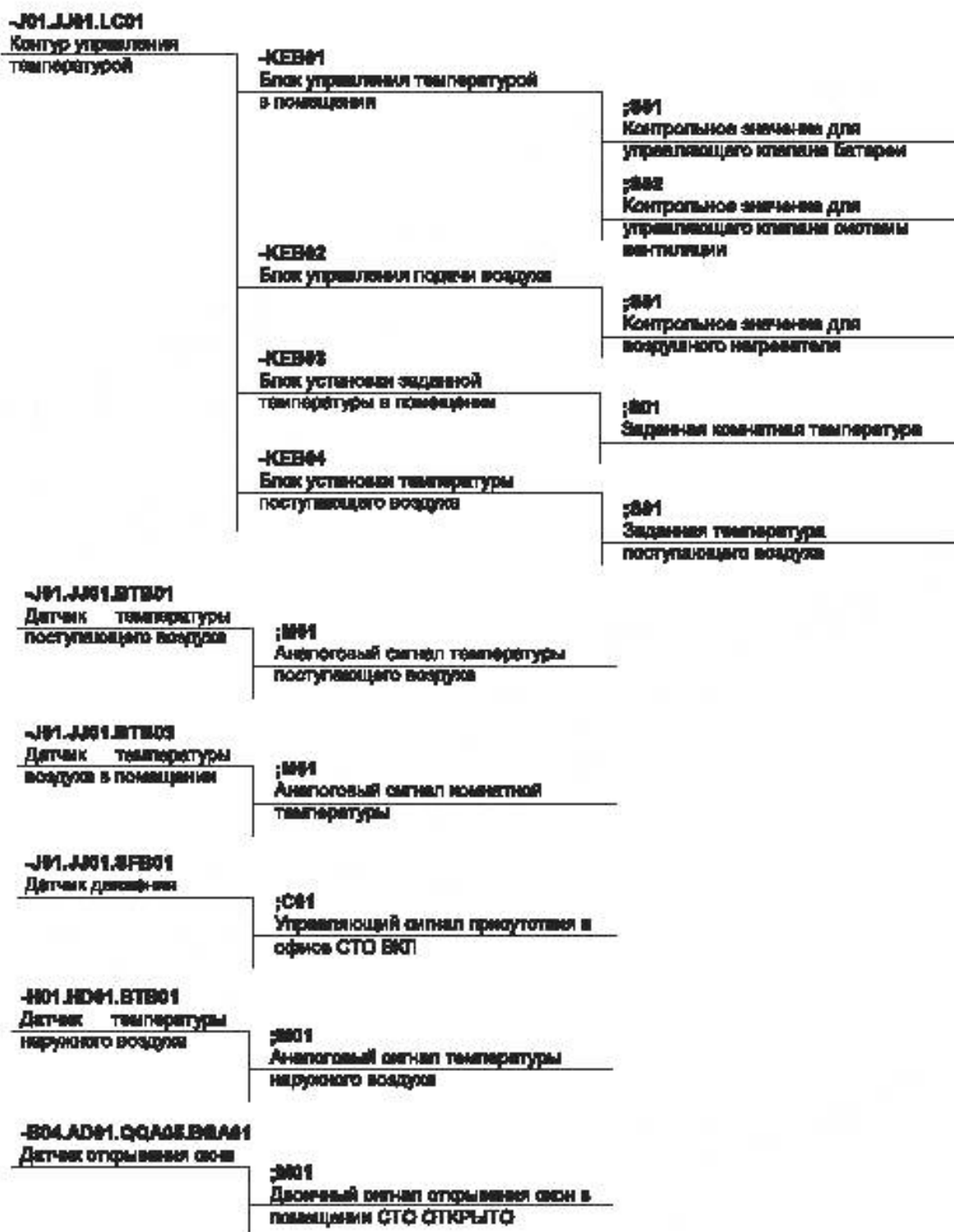
Рисунок В.15 — Древовидная функционально-ориентированная структура представления системы управления инженерными системами помещения (с обозначением системных сигналов)
