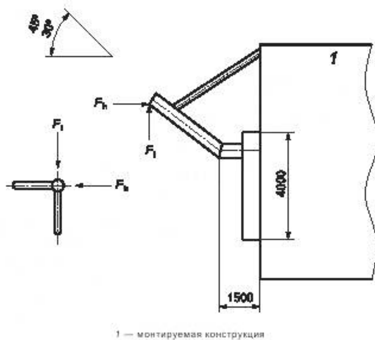
Рисунок А.3 — Горизонтальный рогообразный скользящий кранец с вертикальным направляющим устройством
