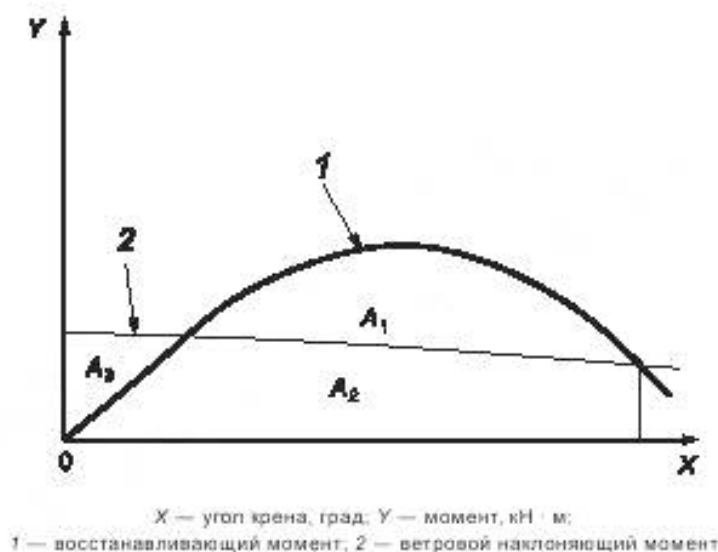
Рисунок 2 — Требование к остойчивости в неповрежденном состоянии
