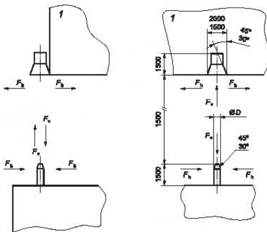
Рисунок А.2 — Направляющий штырь и ловитель
