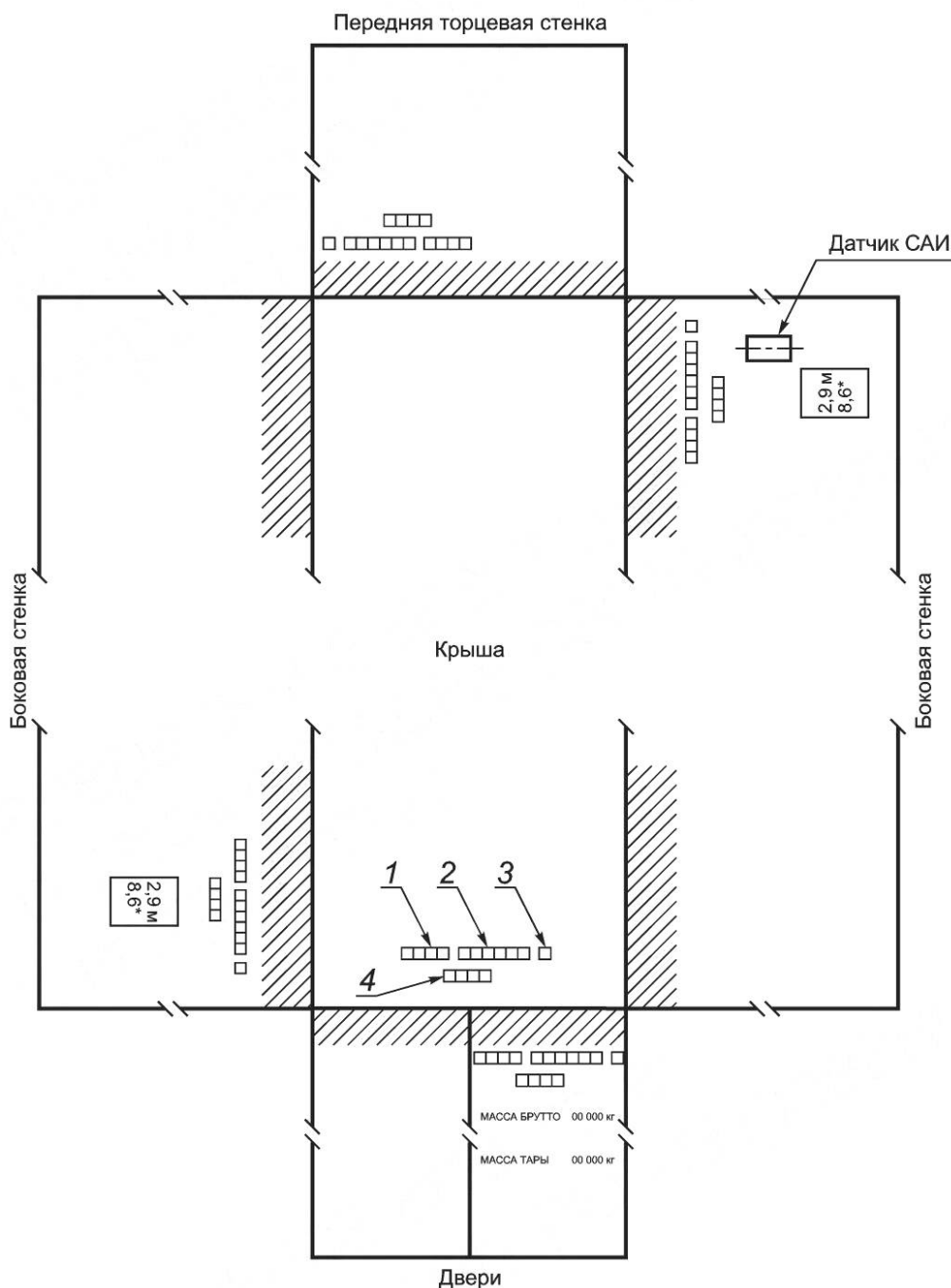
1 — код владельца; 2 — серийный номер; 3 — контрольное число; 4 — код размера и типа Рисунок Б.1 — Схема нанесения маркировки на внешнюю поверхность мобильного (инвентарного) здания
