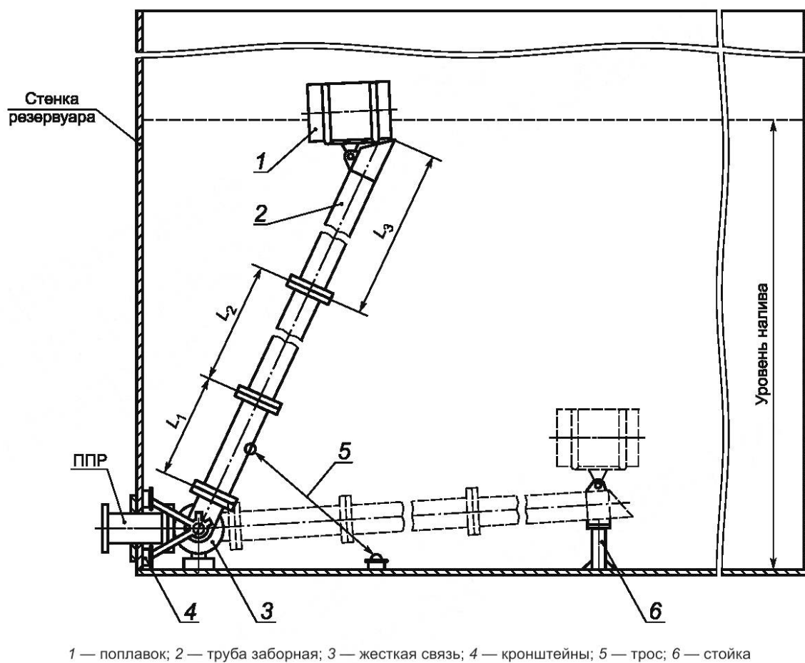
Рисунок А.5 — Общий вид приемо-раздаточного устройства специального типа с плавающим заборным устройством
