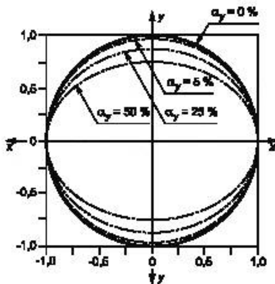
Рисунок А.3 — Влияние разности коэффициентов поглощения образцов на эллипс поляризации излучения после анализатора
