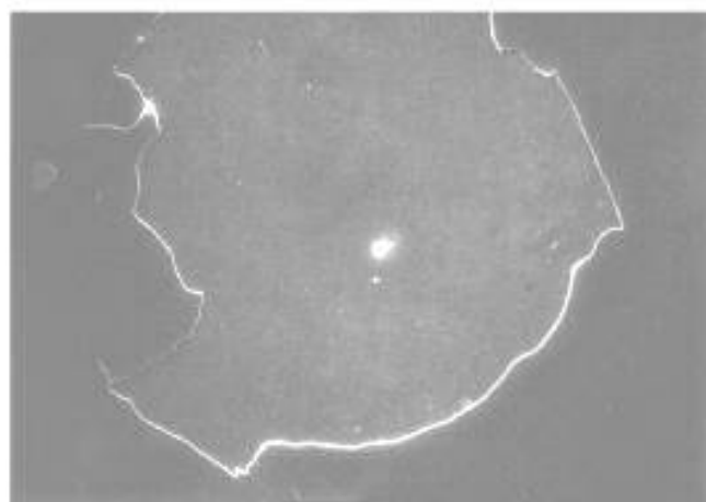
а) 2-слойное просветляющее покрытие (2-QWOT-stack), \text{HfO}_2/\text{SiO}_2 , Nd:YAG-лазер, \tau = 14 нс, E_0 = 45 Дж/см 2 , разрушение, вызванное механическими напряжениями, возникшими в результате поглощения
