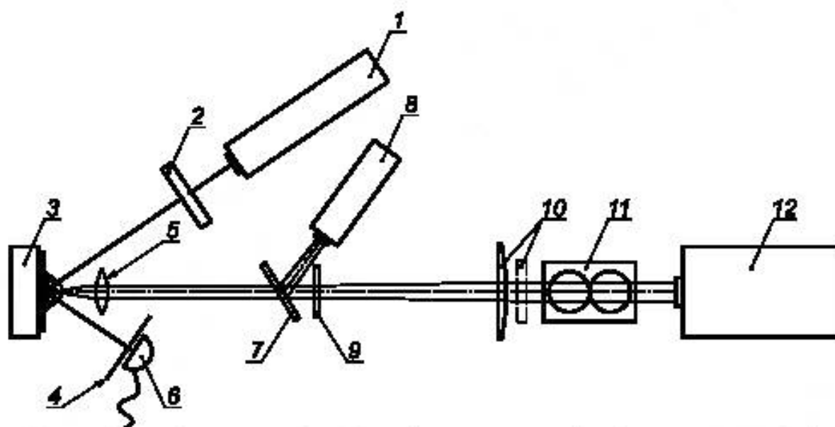
1 — гелий-неоновый лазер; 2 — аттенуатор; 3 — образец; 4 — микроотверстие; 5 — фокусирующая линза; 6 — фотодиод; 7 — светоделитель; 8 — пирометр; 9 — фотошаблон; 10 — томогенизатор и полевая линза; 11 — переменный аттенуатор; 12 — эксимерный лазер
