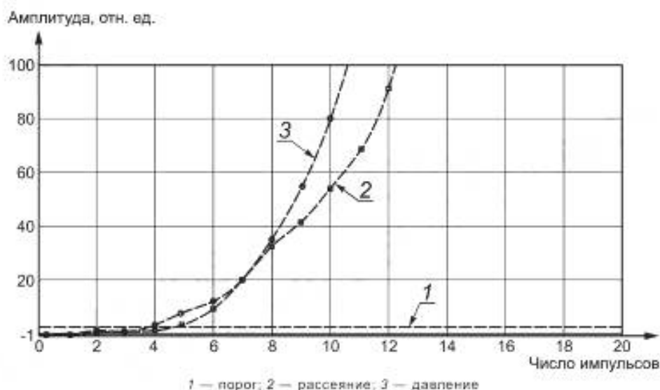
Рисунок 11 — Зависимости величины рассеяния и давления в результате разрушения, возникшего при ~ 4 импульсах для «глухого» зеркала ( \lambda = 1\,064 нм, t_{\text{эфф}} = 3,5 нс, фоновое давление: 4 \times 10^{-6} мбар; f_{\text{и}} = 100 Гц)
