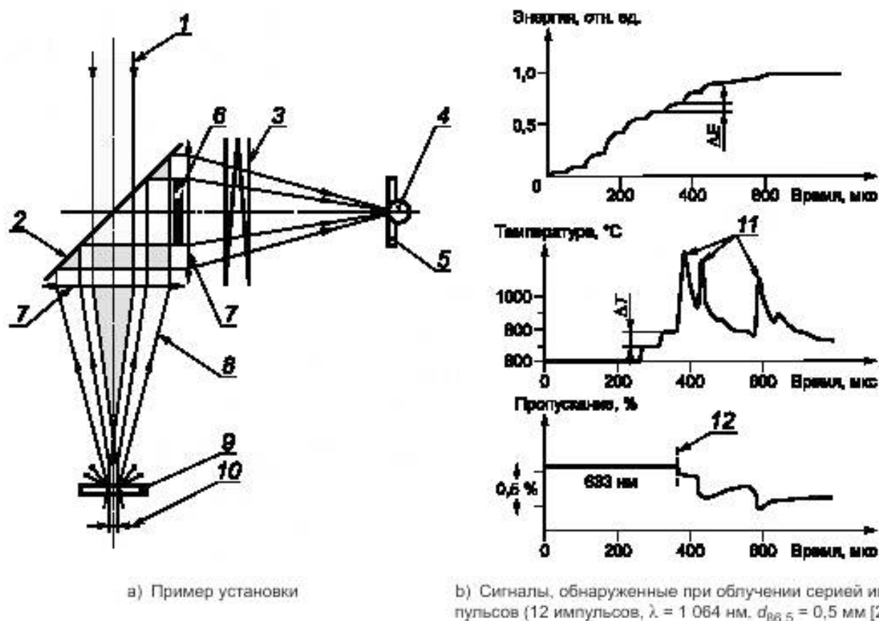
1 — падающий лазерный пучок; 2 — дихроичный расщепитель пучка HT 1060/HR 850/45°; 3 — набор фильтров HT 850/HR 1060; 4 — кремниевый фотодиод; 5 — диафрагма, настроенная на размер пятна; 6 — поле рассеяния; 7 — фокусирующая линза; 8 — излучение, характеризующее температуру; 9 — образец; 10 — размер пятна; 11 — плазма; 12 — разрушение
