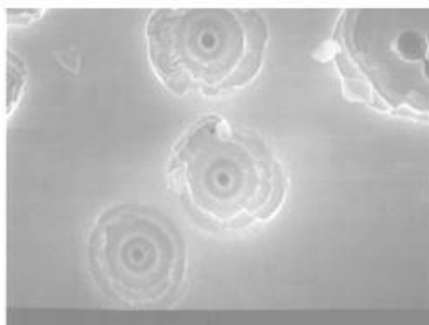
б) однослойное просветляющее покрытие, пленка \text{HfO}_2/\text{SiO}_2 , Nd:YAG-лазер, \tau = 14 нс, разрушение, вызванное дефектами
