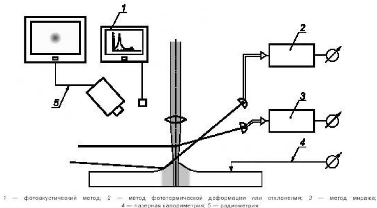
Рисунок 7 — Схемы фототермических измерений
