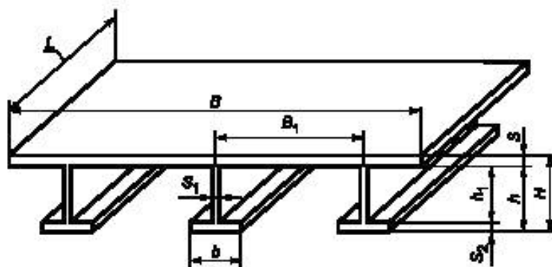
L — длина панели; B — ширина панели; B_1 — межреберное расстояние; S — толщина полотна панели; H — высота панели; h — высота ребра; h_1 — высота ножки ребра; b — ширина полки (бульбы) ребра; S_1 — толщина ножки ребра; S_2 — толщина полки ребра
