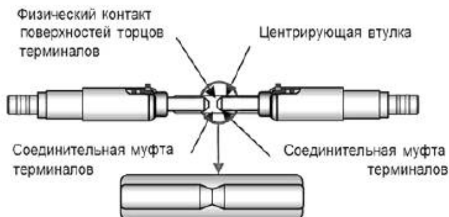
Рисунок 1 — Интерфейс и центровка волоконно-оптических терминалов
