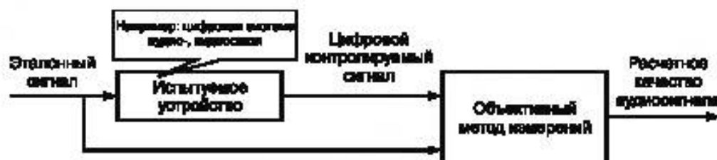
Рисунок 8 — Базовая модель проведения объективных измерений
