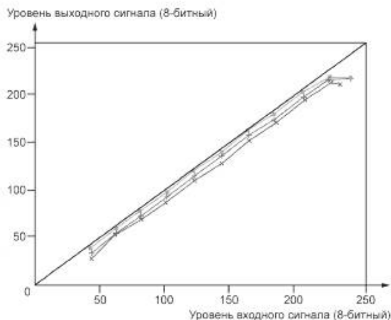
Рисунок 4 — Пример графика воспроизведения тонов
