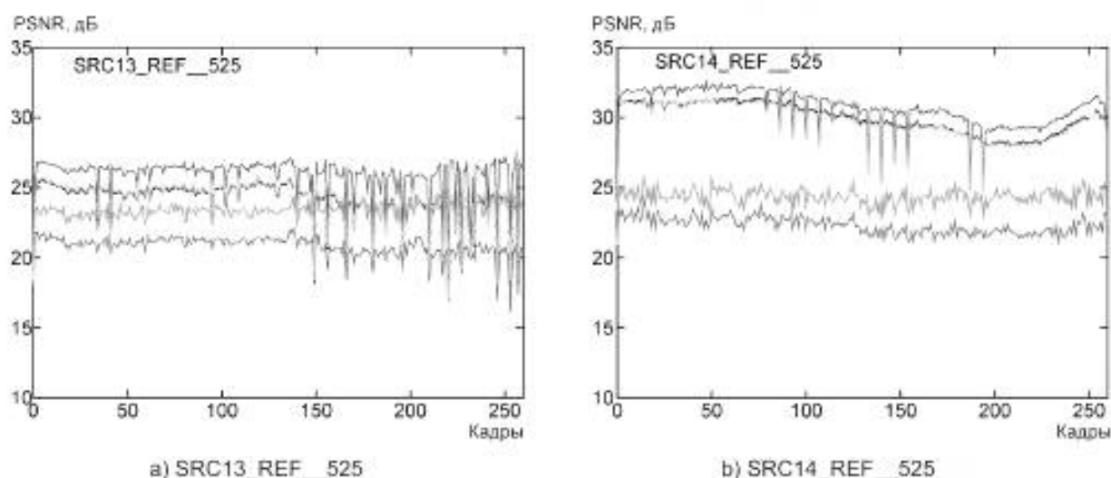
Рисунок 7 — Примеры оценки PSNR, лист 1
