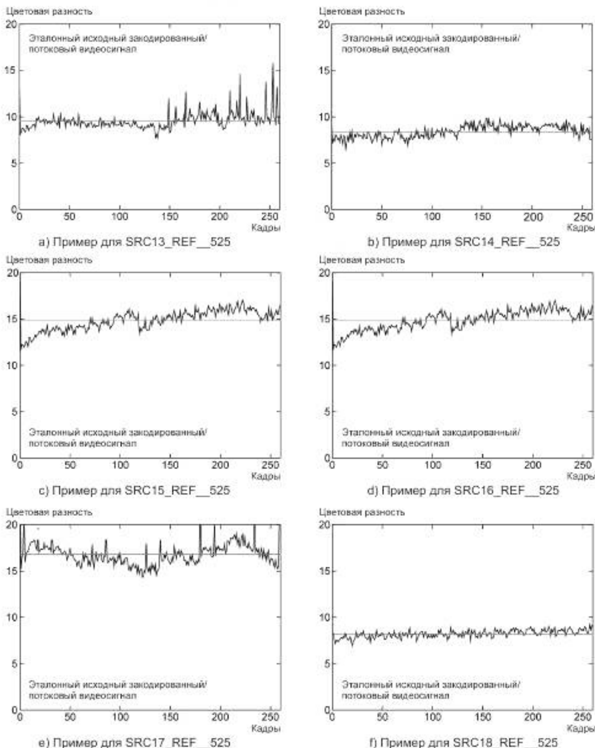
Рисунок 6 — Цветовые разности между эталонными и потоковыми видеок кадрами при 250 кбит/с и 30 кадр/с, лист 1
