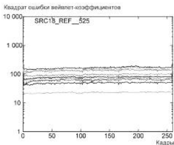
Рисунок В.3 — Диаграммы разности коэффициентов вейвлет-преобразования между эталонным и потоковым видеокдрами при скорости 250 кбит/с и 30 кадр/с, лист 1
