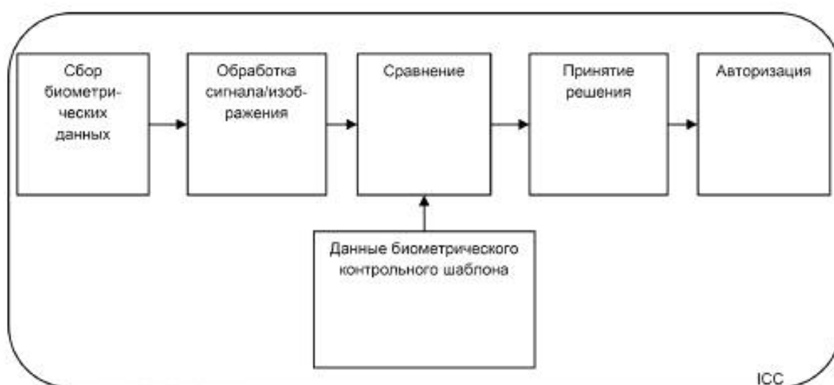
Рисунок 4 — Общая архитектура для биометрического распознавания с использованием сравнения на идентификационной карте
