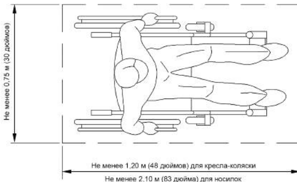
Рисунок А.1 — Чистая площадь пола
