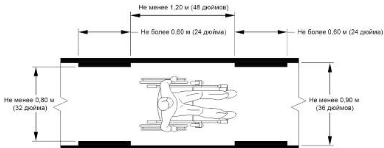
Рисунок А.2 — Свободная ширина прохода
