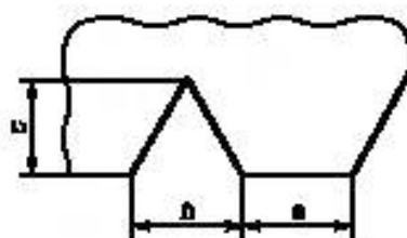
Рисунок А.1 — Форма вырезов зубчатых шпателей
