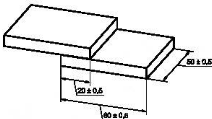
Рисунок 2 — Образец клеевого соединения при испытании на сдвиг
