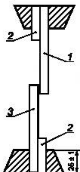
1 — не покрытое клеем основание; 2 — уплотнитель; 3 — покрытие
