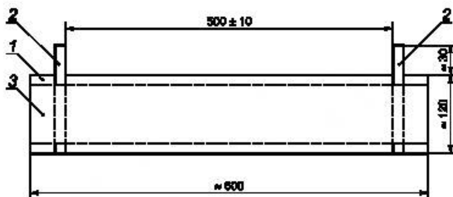
1 — плита стеклянная; 2 — пластина медная; 3 — клеевой слой
