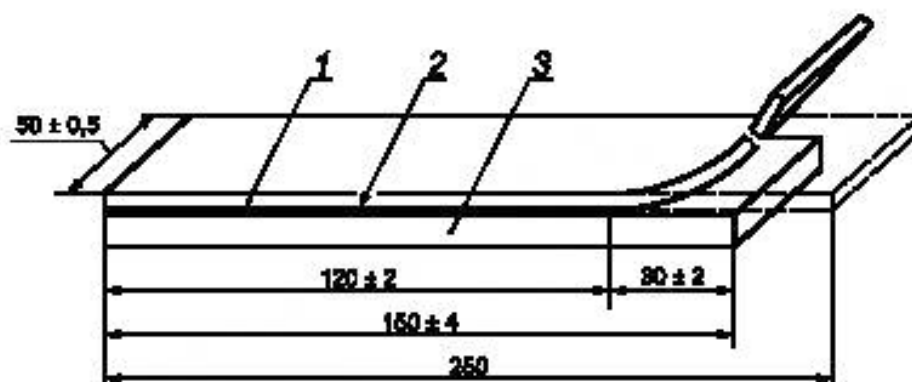
1 — испытываемое покрытие; 2 — клей; 3 — основание
