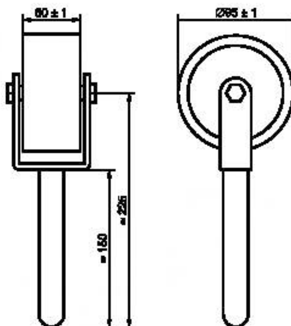
Рисунок 1 — Каток ручной
