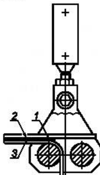
1 — основание; 2 — клей; 3 — испытуемое покрытие
