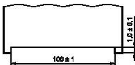
Рисунок 9 — Схема аппликатора для нанесения клея
