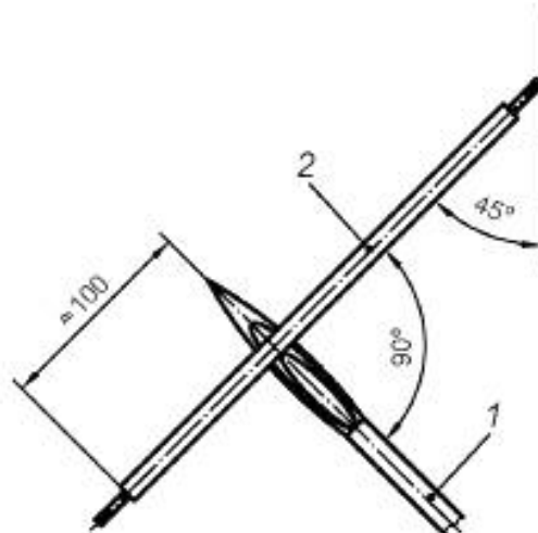
1 — горелка Бунзена; 2 — образец
