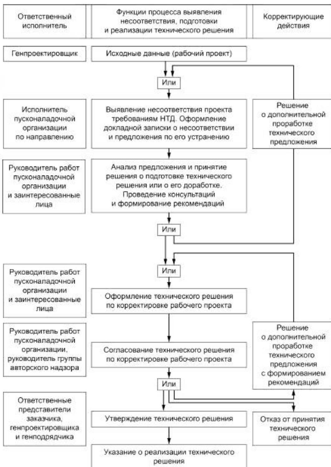
Рисунок В.1 — Алгоритм внесения изменений в рабочую документацию
