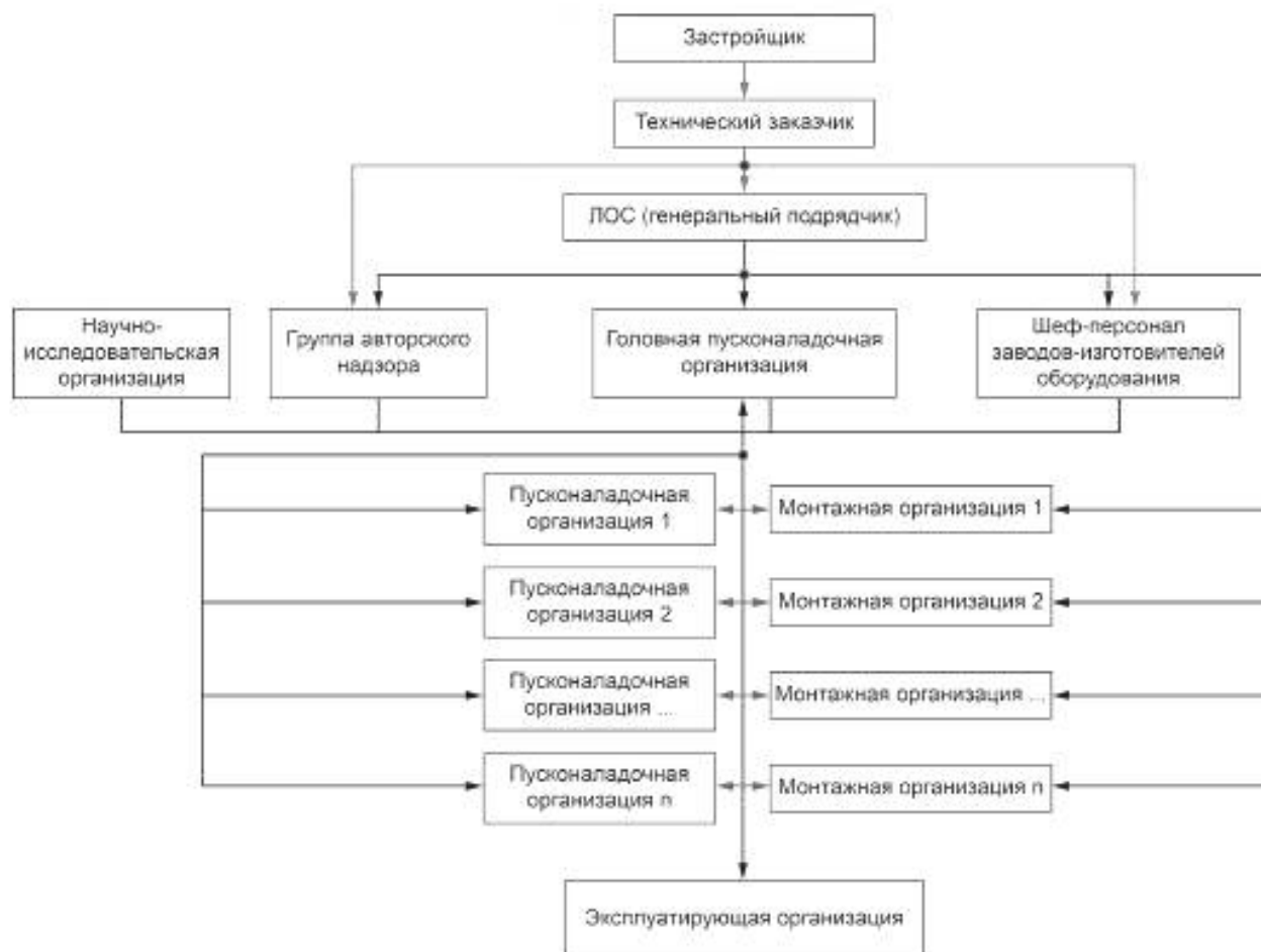
Рисунок А.1 — Форма организационной структуры производства пусконаладочных работ
