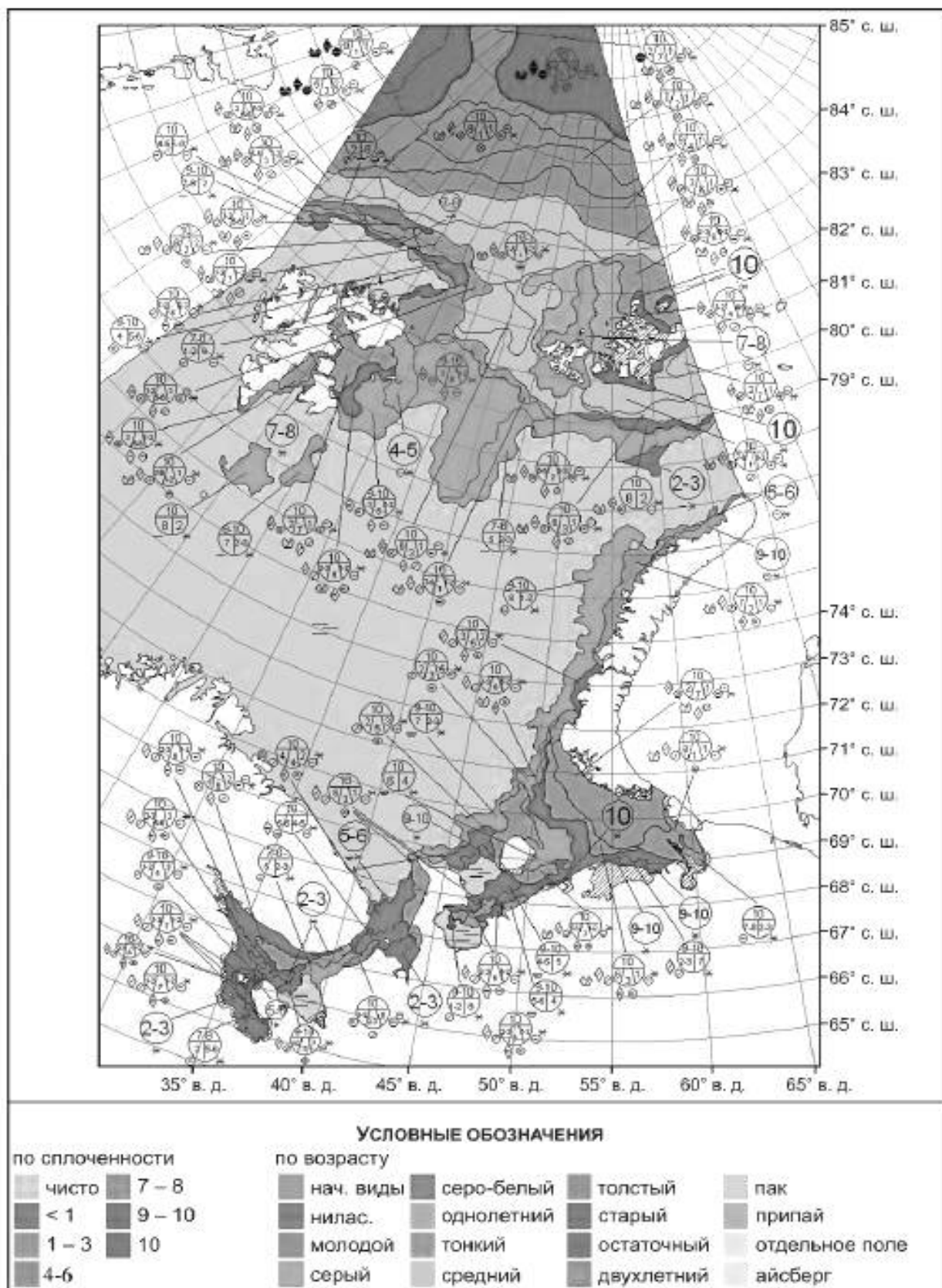
Рисунок Б.2 — Пример генерализованной карты состояния ледяного покрова
