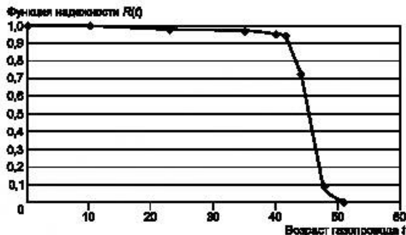
Рисунок Б.1 — График эмпирической функции надежности R(t)
