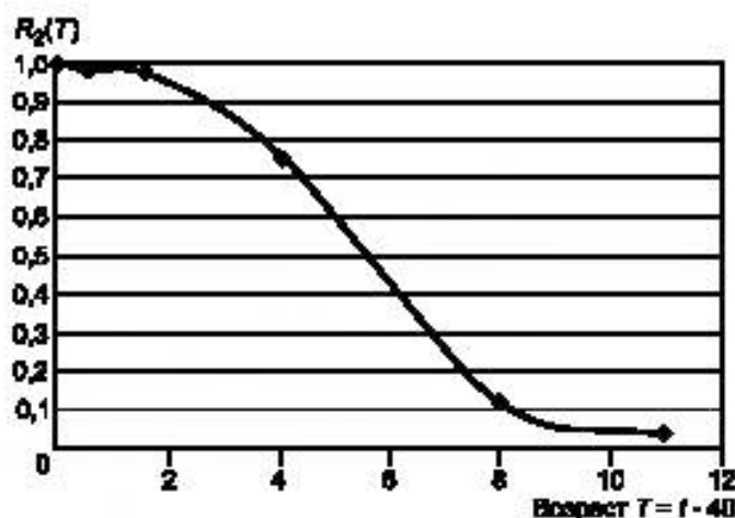
Рисунок Б.2 — Эмпирическая функция надежности R_2(T)
