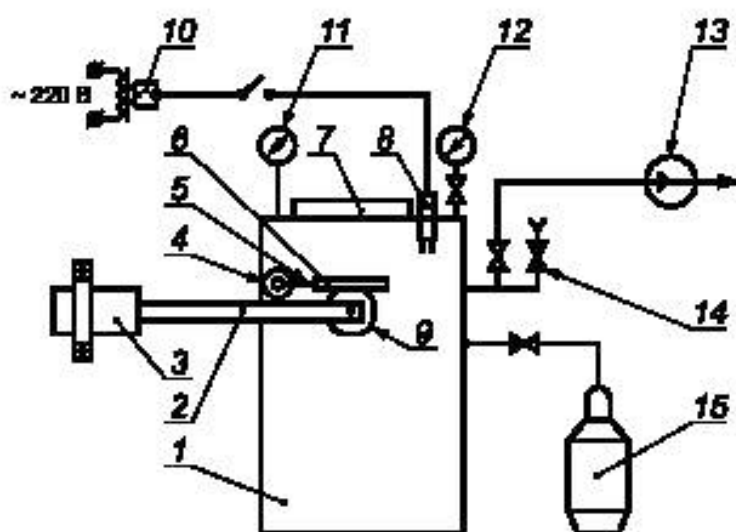
1 — реакционный сосуд; 2 — передаточный механизм; 3 — электродвигатель; 4 — прижимной механизм; 5 — держатель; 6 — пластина; 7 — крышка; 8 — свеча; 9 — вращающийся диск; 10 — понижающий трансформатор; 11 — манометр; 12 — вакуумметр; 13 — вакуумный насос; 14 — вентиль; 15 — баллон с горючим газом
