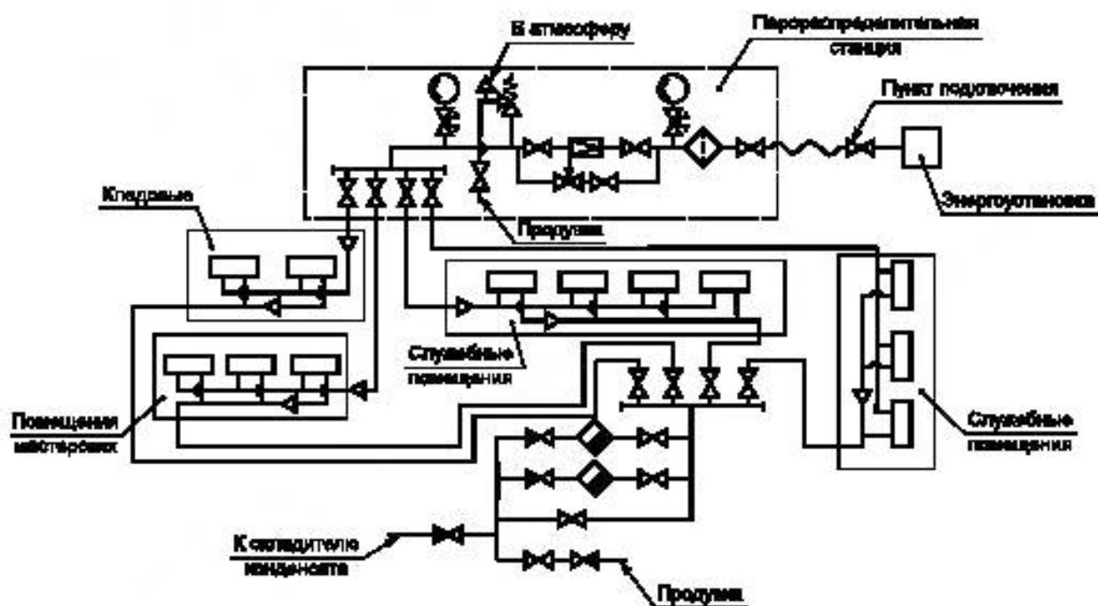
Рисунок Б.2 — Типовая схема двухпроводной проточной СПО
