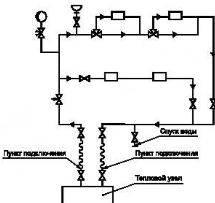
Рисунок Б.5 — Типовая схема однопроводной СЖО
