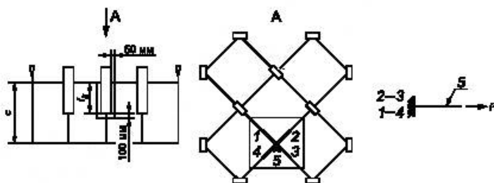
1—4 — расположение образца при отборе из геомодуля и проведении испытаний (обозначения 1, 4 и 2, 3 относятся к одному образцу); 5 — расположение монтажной проушины; P — нагрузка на образец; s — высота ячейки; L_k — высота крепления монтажной проушины к ячейке геомодуля
