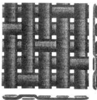
Рисунок 3 — Углеродная ткань сатинового переплетения
