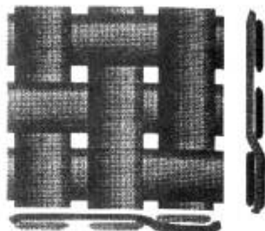
Рисунок 2 — Углеродная ткань саржевого переплетения
