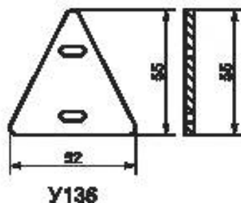
Рисунок 2 — Бирка пластиковая для маркировки информационно-питающих кабелей (напряжение питания до ~ 80 В)
