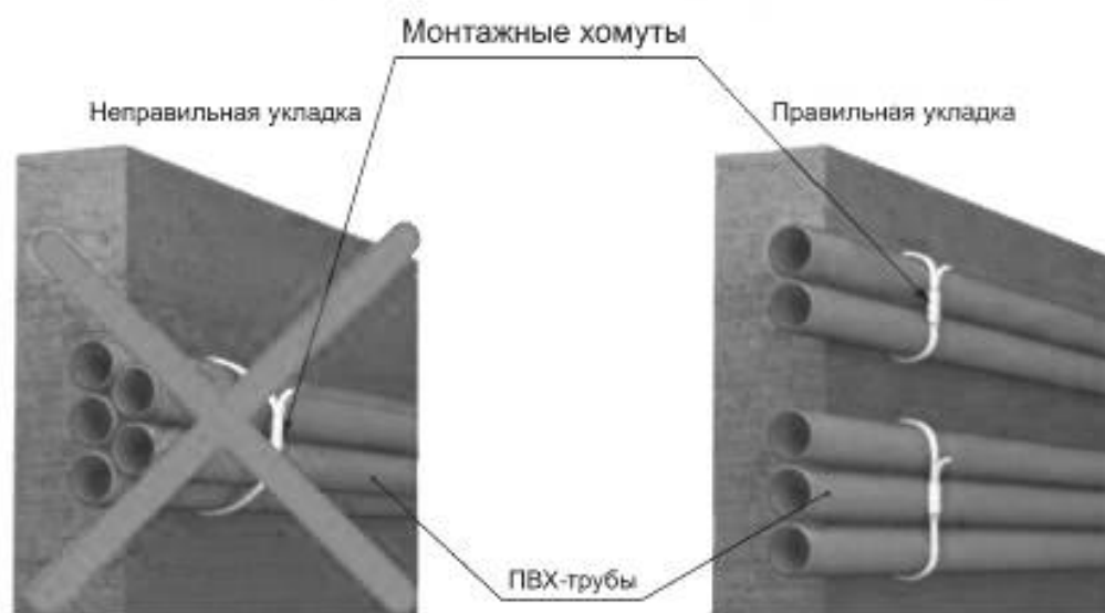
Рисунок 1 — Правило укладки пластиковых труб в пакеты
