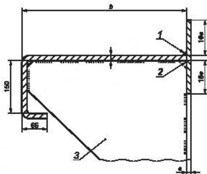
е) Гнутый лист
