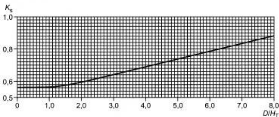
Рисунок G.3 — Коэффициент K_s
