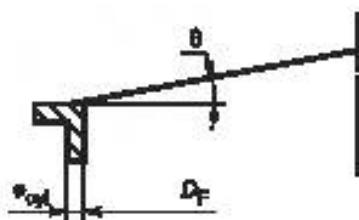
Рисунок К.1 — Коническая крыша
