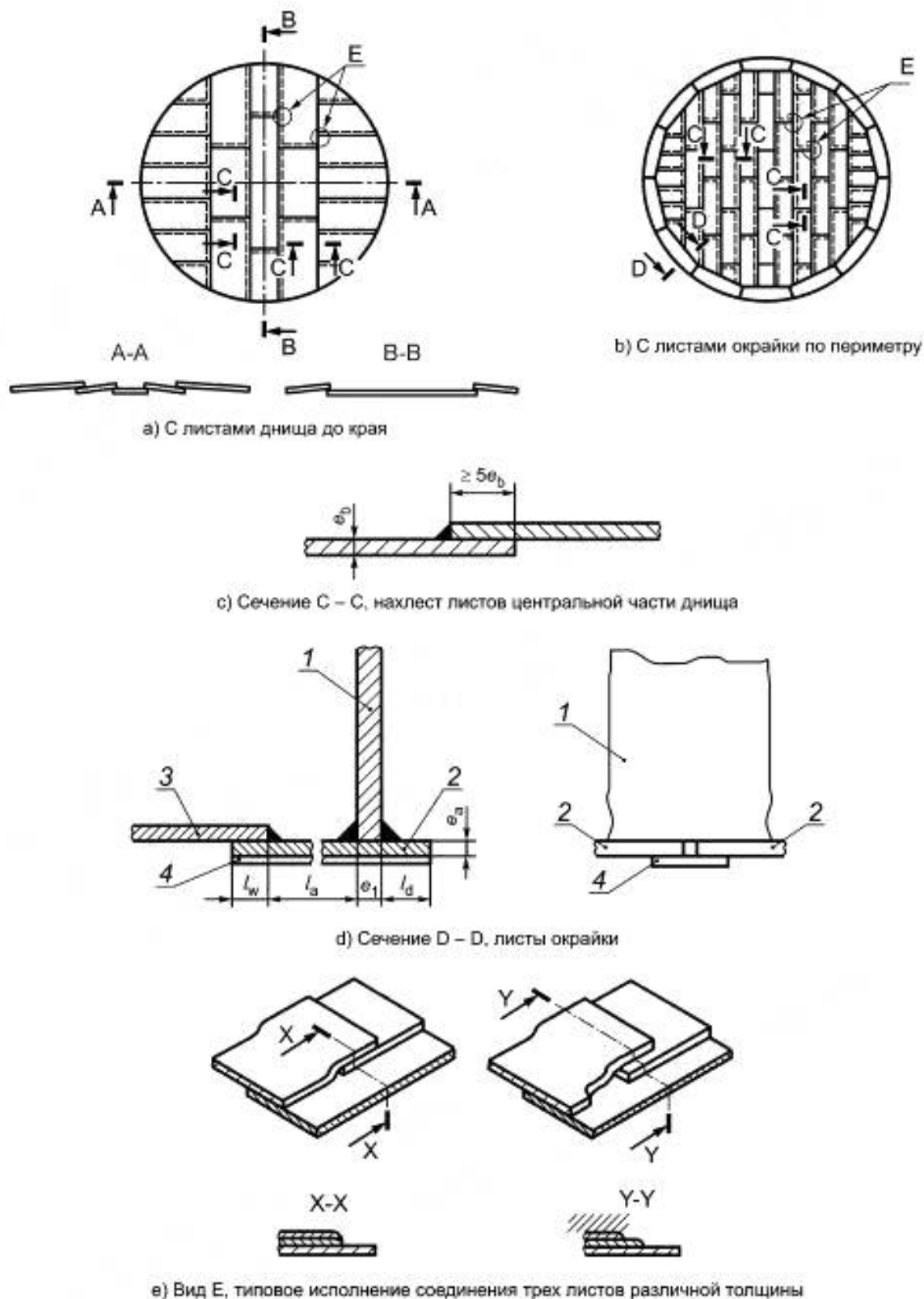
Рисунок 3 — Типовые конструкции дна резервуара
