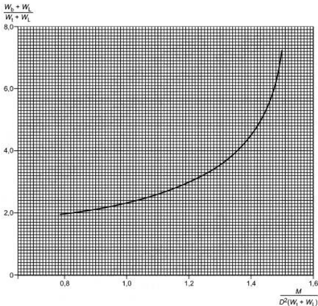
Рисунок G.4 — Усилие сжатия W_b
