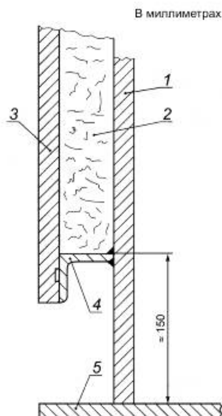
Рисунок Q.4 — Типовое примыкание теплоизоляции в области дна резервуара
