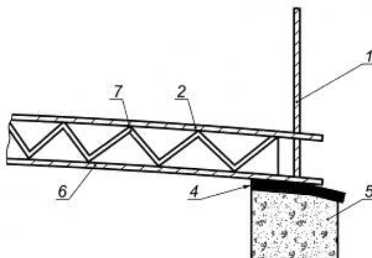
б) Двойное днище, разделенное решеткой из стали
