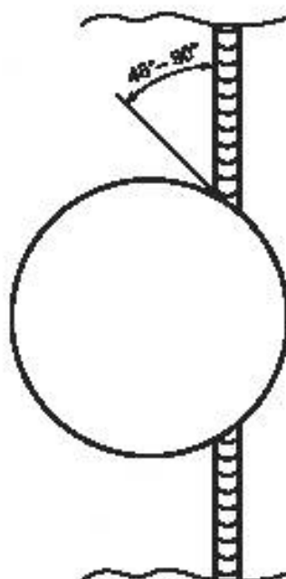
Рисунок 17 — Отверстия для патрубков, пересекающих швы стенки
