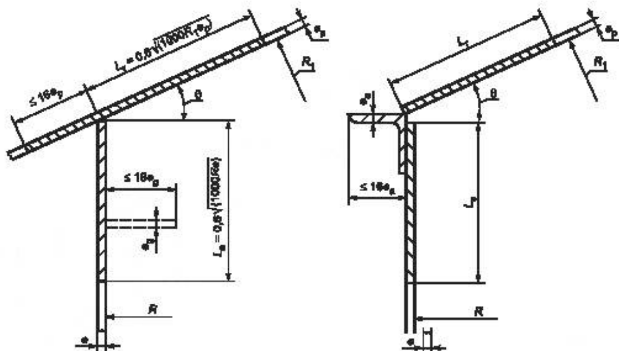
а) Без опорного кольца из углового профиля
