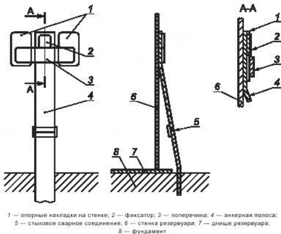
Рисунок М.1 — Типовое исполнение анкерной полосы
