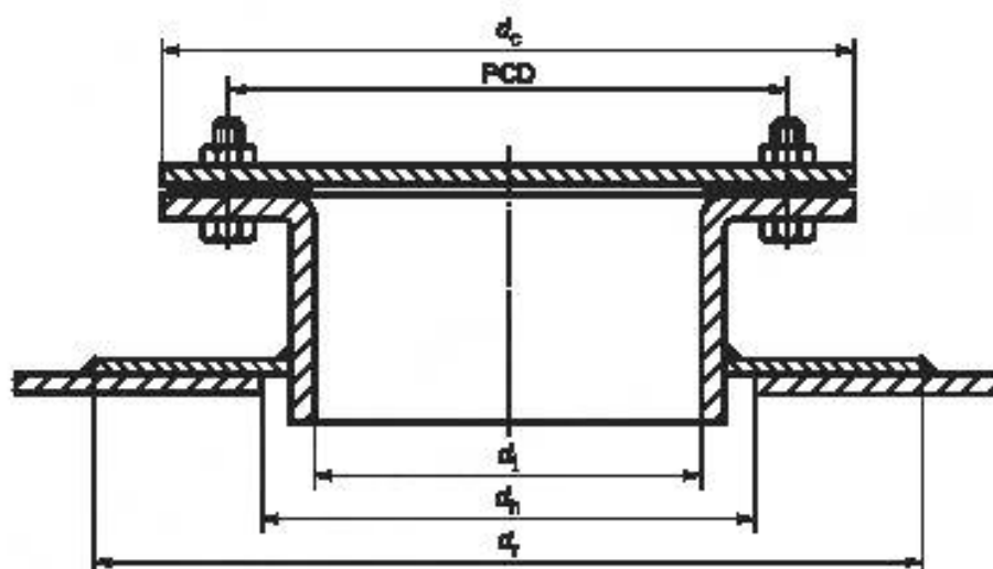
Рисунок 15 — Крышка на болтах
