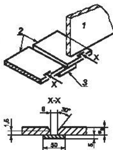
1 — лист стенки; 2 — листы окрайки; 3 — подкладная полоса
