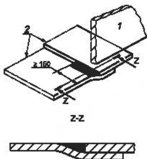
1 — лист стенки; 2 — лист дна в краевой части
