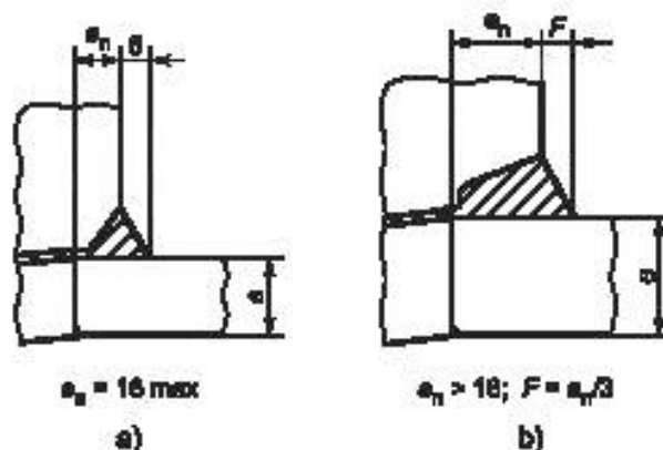
Рисунок N.2 — Типовые исполнения накладных патрубков, привариваемых встык
