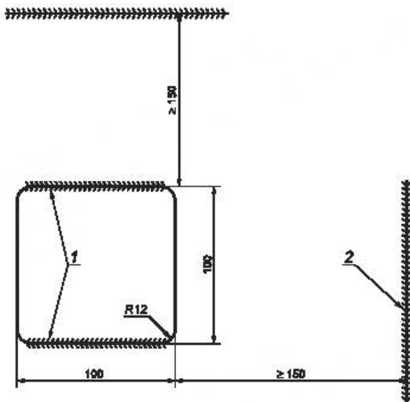
Рисунок Q.1 — Крепежные пластины
