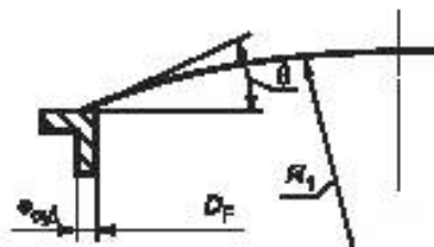
Рисунок К.2 — Сферическая крыша
