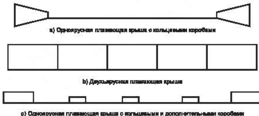
Рисунок D.1 — Типовые примеры плавающих крыш
