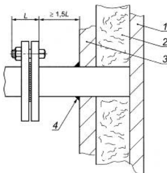
1 — стенка резервуара; 2 — теплоизоляция; 3 — обшивка; 4 — герметик
