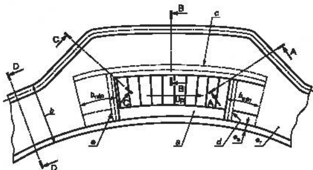
Рисунок 7 — Лестница, проходящая сквозь кольцо жесткости
