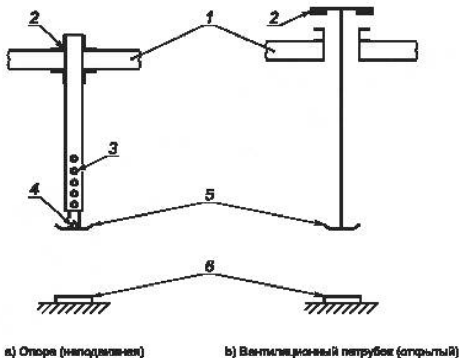
1 — понтон; 2 — уплотнитель; 3 — резьбовые отверстия для регулировки высоты; 4 — сливное отверстие; 5 — опорная плита; 6 — усиливающая накладка
