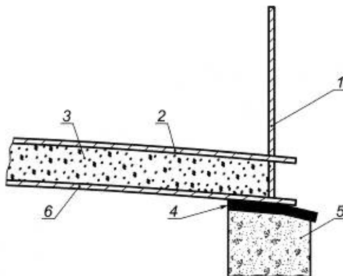
а) Двойное днище с пористым заполнением
