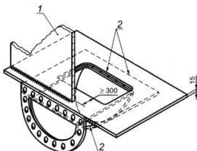
Рисунок 0.5 — Типовое исполнение зумпфов резервуаров
