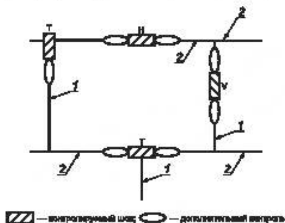
Рисунок 19 — Дополнительный контроль дефектных швов
