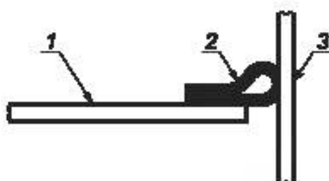
б) Петлевой затвор
