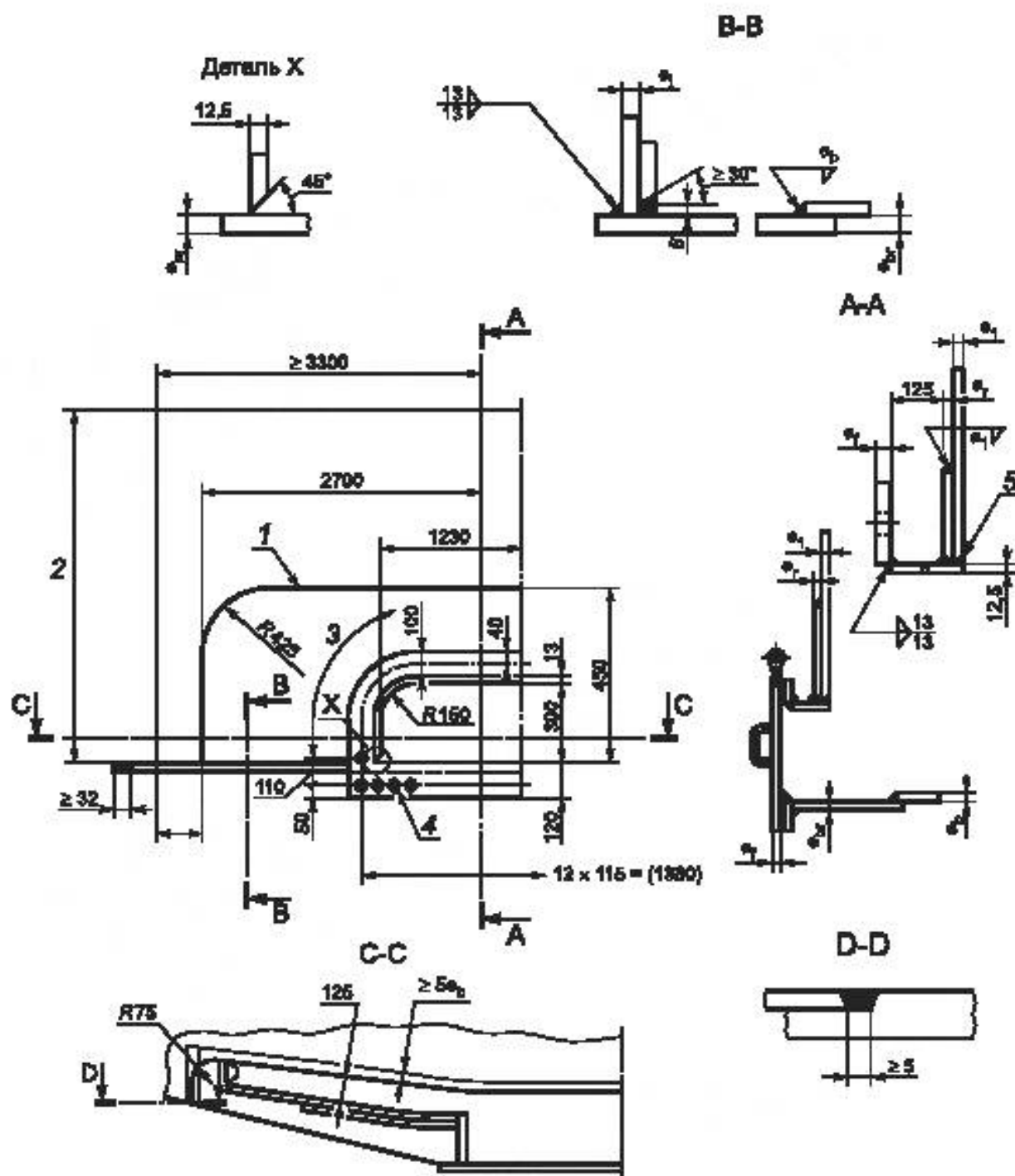
1 — усиливающий лист; 2 — высота врезки; 3—20 равных расстояний; 4 — 34 отверстия Ø 28 для болтов М24; 5 — сварной шов [см. рисунок 11 б)]; e_1 — толщина стенки нижнего пояса; e_1 — толщина врезки; e_2 — толщина крышки и фланца; e_{1\Gamma} — толщина усиливающего листа днища; e_6 — толщина листа днища
