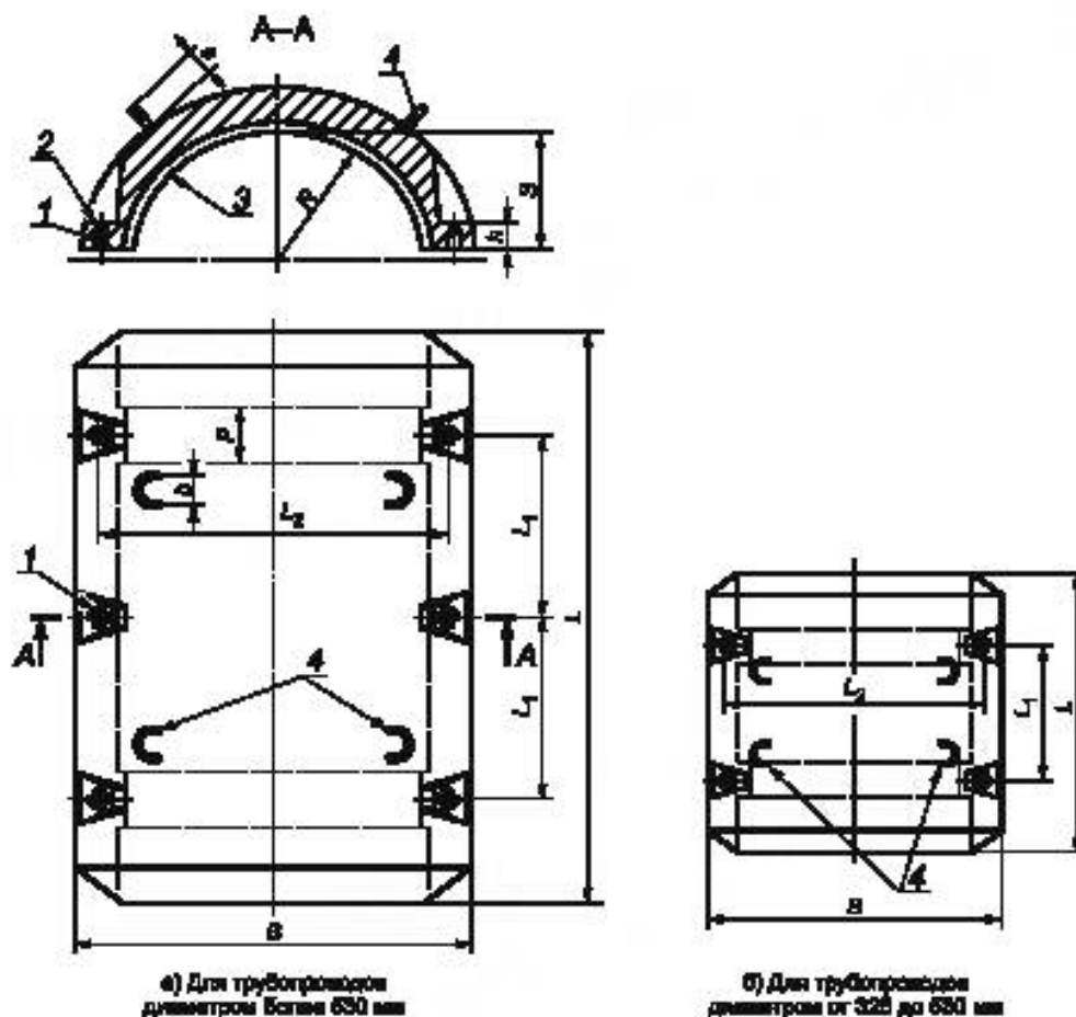
Рисунок 1 — Общий вид полугрузов кольцевого балластирующего устройства
