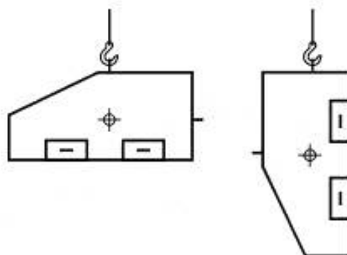
Рисунок 3 — Положение БУОТ на подвеске ( — положение \oplus проекции центра масс на боковой грани БУОТ)
