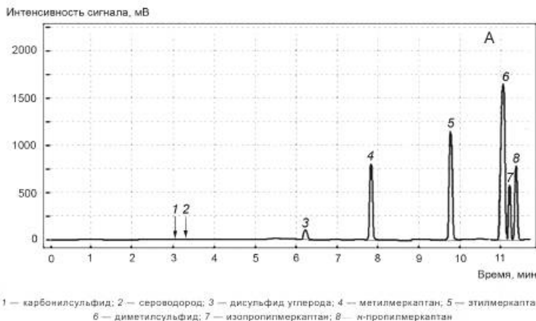
Рисунок Б.8 — Хроматограмма серосодержащих соединений нестабильного газового конденсата (канал В), полученная на капиллярной колонке в режиме программирования температуры с детектированием на ПФД (при условиях, приведенных в таблице 6 настоящего стандарта) (фрагмент А)
