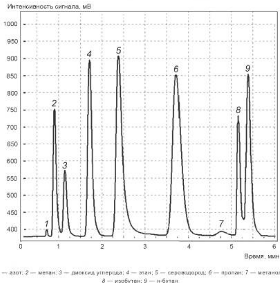
Рисунок Б.1 — Хроматограмма нестабильного газового конденсата (канал А), полученная на насадочной колонке (Porapak Q) при изотермическом режиме с детектированием на ДТП (условия хроматографического разделения приведены в таблице 4 настоящего стандарта)
