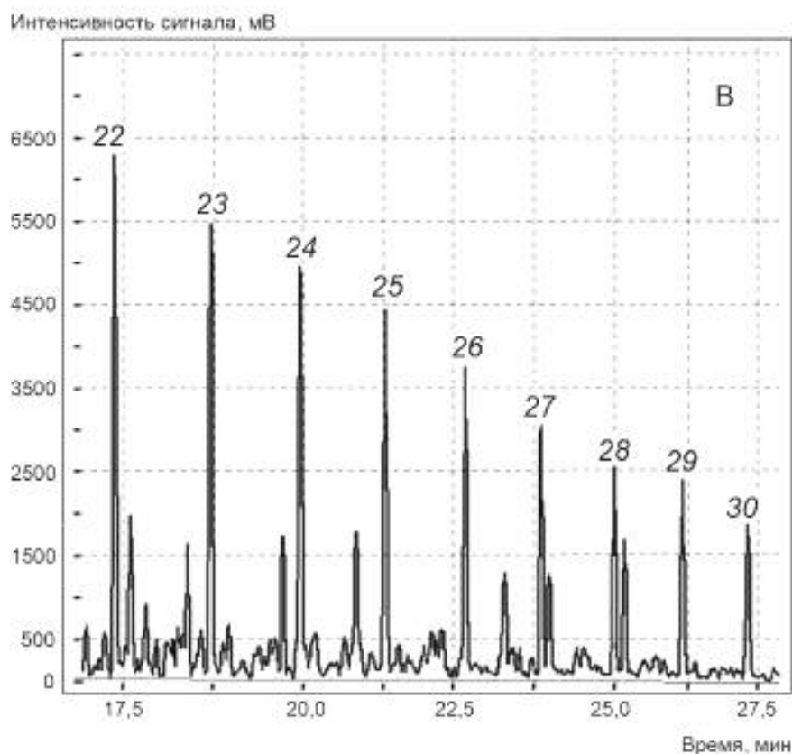
Рисунок Б.4 — Хроматограмма нестабильного газового конденсата (канал Б), полученная на капиллярной колонке в режиме программирования температуры с детектированием на ПИД (условия хроматографического разделения приведены в таблице 5 настоящего стандарта) (фрагмент В)
