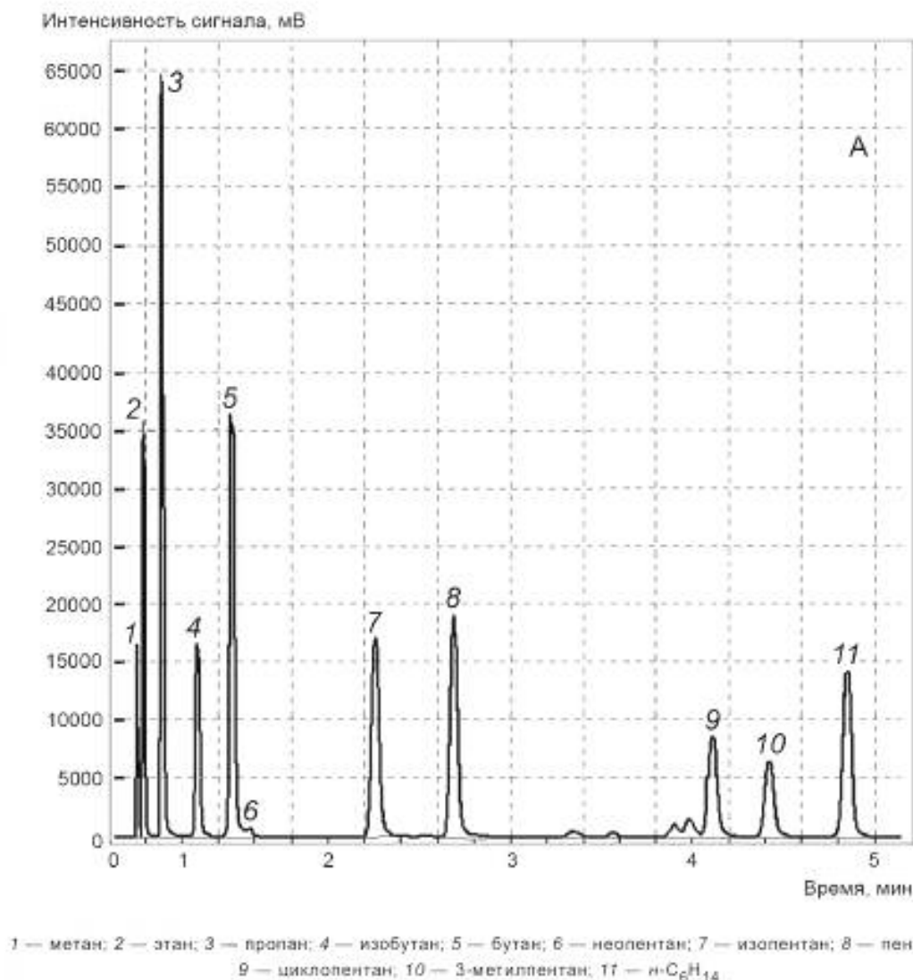
Рисунок Б.2 — Хроматограмма нестабильного газового конденсата (канал Б), полученная на капиллярной колонке в режиме программирования температуры с детектированием на ПИД (условия хроматографического разделения приведены в таблице 5 настоящего стандарта) (фрагмент А)
