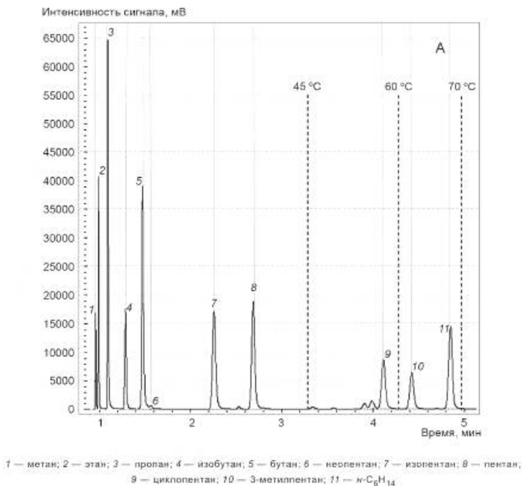
Рисунок Д.3 — Пример разметки хроматограммы углеводородов нестабильного газового конденсата на фракции, сформированные по температурам кипения (фрагмент А)
