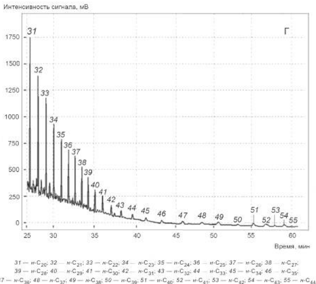
Рисунок Б.5 — Хроматограмма нестабильного газового конденсата (канал Б), полученная на капиллярной колонке в режиме программирования температуры с детектированием на ПИД (условия хроматографического разделения приведены в таблице 5 настоящего стандарта) (фрагмент Г)
