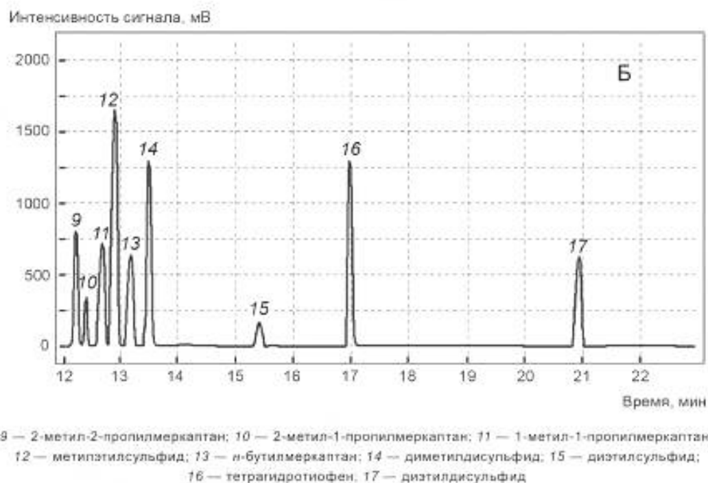
Рисунок Б.9 — Хроматограмма серосодержащих соединений нестабильного газового конденсата (канал В), полученная на капиллярной колонке в режиме программирования температуры с детектированием на ПФД (при условиях, приведенных в таблице 6 настоящего стандарта) (фрагмент Б)
