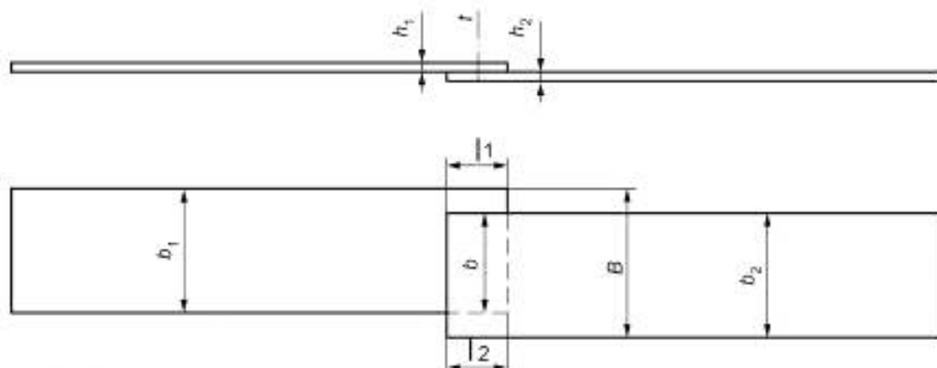
Рисунок 4 — Схема замера образца
