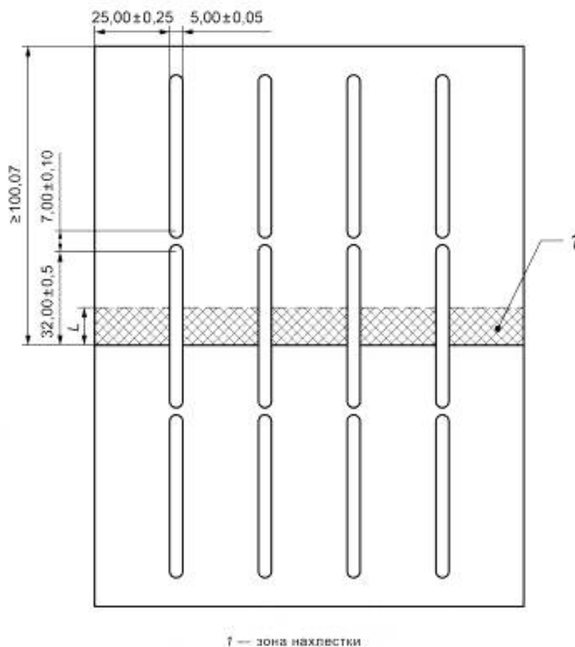
Рисунок 3 — Панель с прорезями для изготовления образцов (только для приемочных испытаний)
