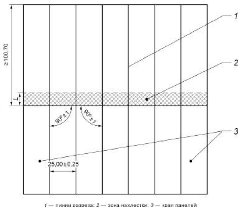
Рисунок 2 — Стандартная панель для изготовления образцов
