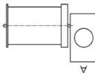
б) лебедка правого исполнения с односекционным барабаном
