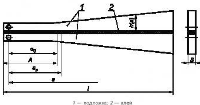
Рисунок 4 — Образец для испытания методом КДКБ
