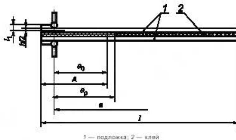
Рисунок 2 — Образец для испытания методом ДКБ с петлями (альтернативный режим нагружения)
