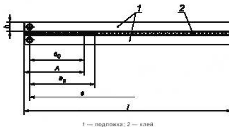
Рисунок 3 — Образец для испытания методом ДКБ с металлическими подложками и высверленными отверстиями (альтернативный режим нагружения)
