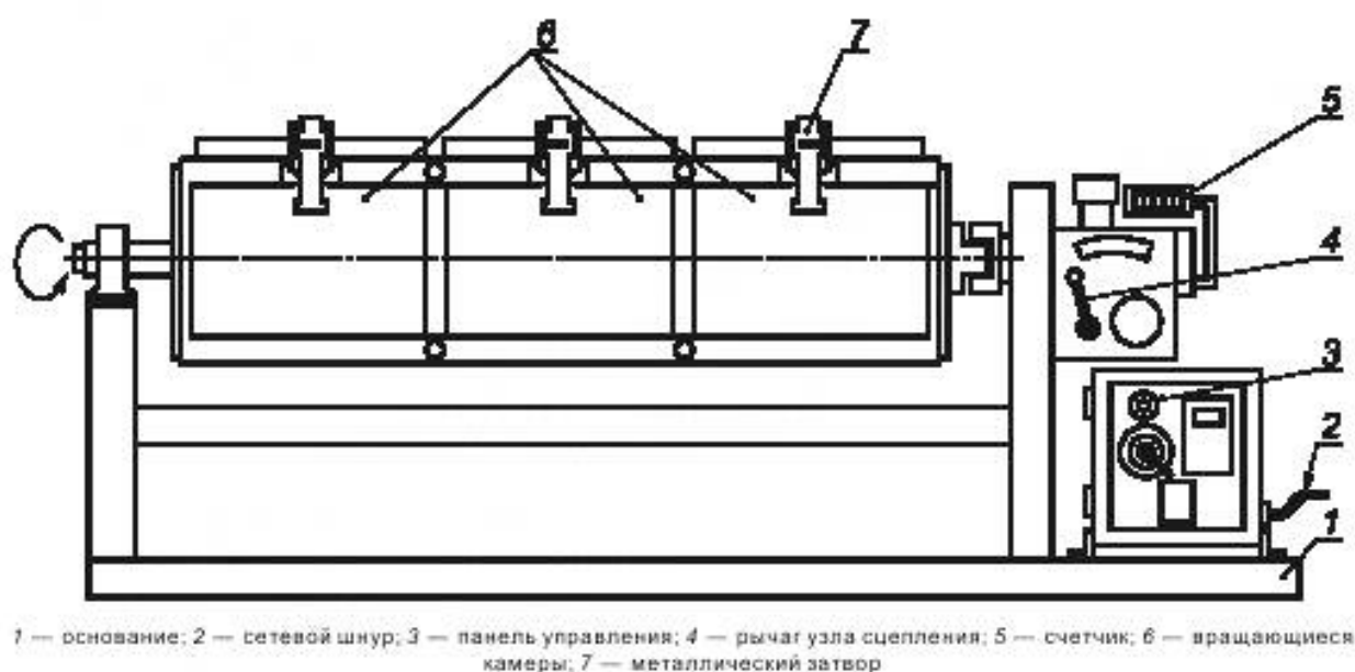
Рисунок А.1 — Схема прибора типа ICI Pilling Tester (компоновка узлов прибора других модификаций может отличаться от приведенной на схеме)
