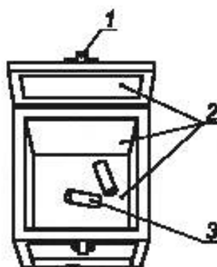
Рисунок А.1 — Схема прибора типа ICI Pilling Tester (компоновка узлов прибора других модификаций может отличаться от приведенной на схеме)
