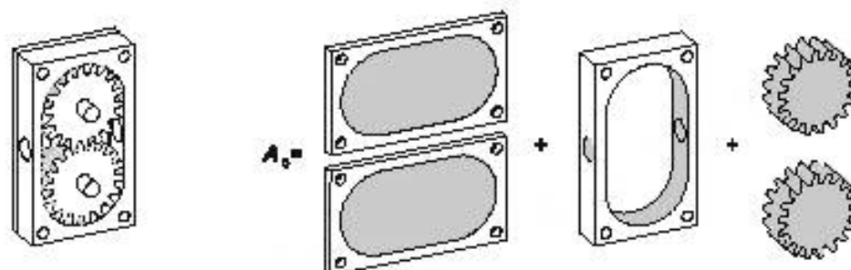
Рисунок 1 — Смачиваемая поверхность механизма внешнего гидравлического насоса
