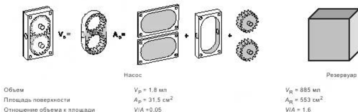
Рисунок С.1 — Насос с зубчатой передачей внешнего сцепления и резервуар
