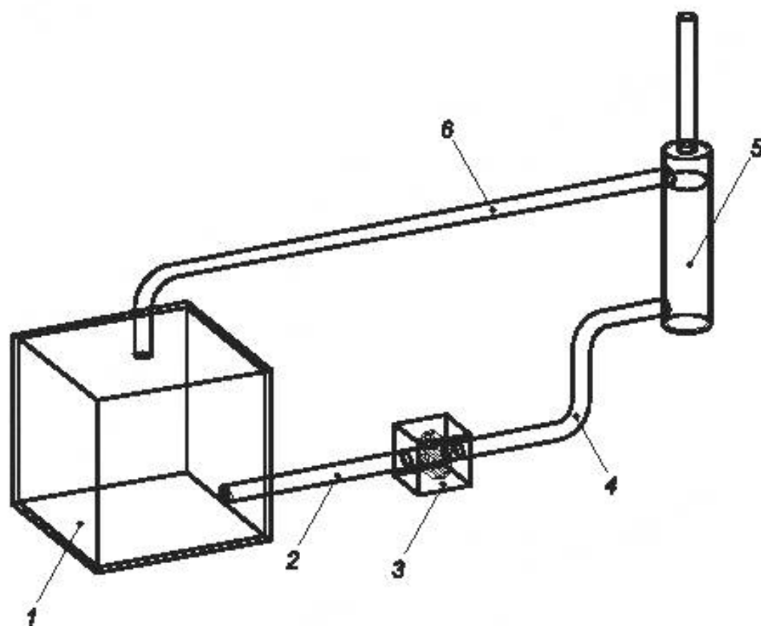
Рисунок В.1 — Упрощенный гидравлический контур
