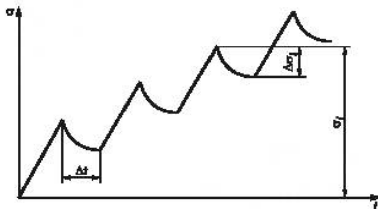
Рисунок 3 — Кривая зависимости напряжения от времени
