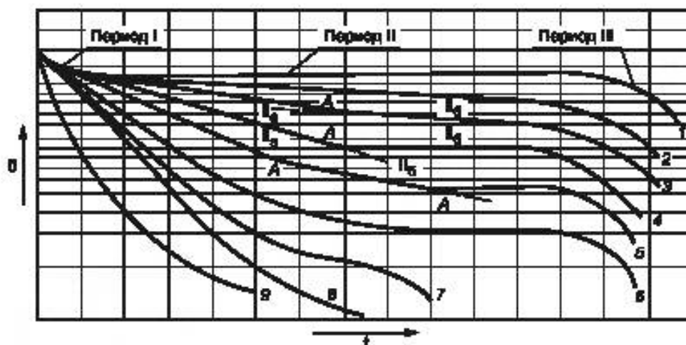
Рисунок 1 — Типовые кривые релаксации в координатах «напряжение — время»
