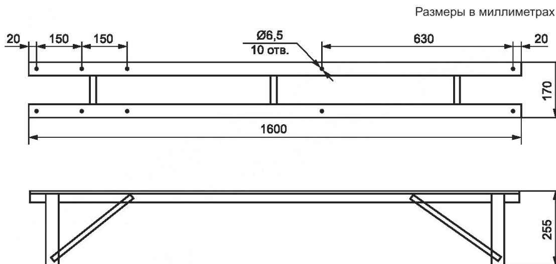
Рисунок Б.3 — Подставка для закрепления образца».
